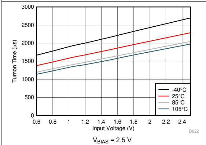
图 6-27. Turnon Time vs Input Voltage
