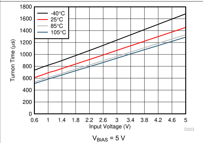
图 6-28. Turnon Time vs Input Voltage
