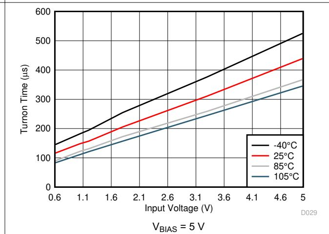
图 6-42. Turnon Time vs Input Voltage
