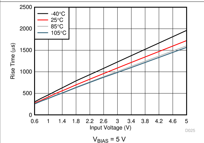
图 6-30. Rise Time vs Input Voltage
