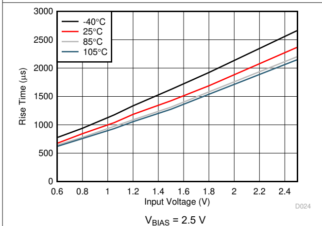
图 6-29. Rise Time vs Input Voltage
