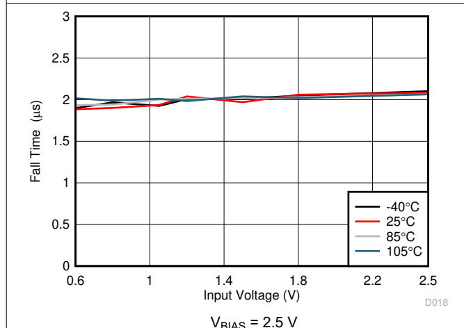
图 6-21. Fall Time vs Input Voltage
