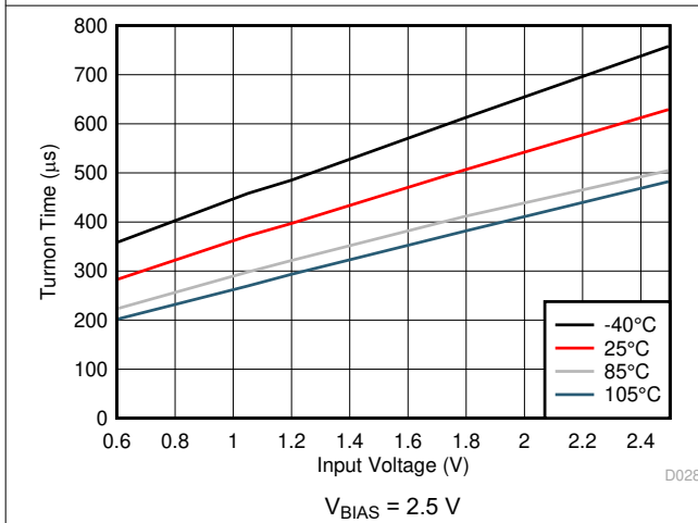
图 6-41. Turnon Time vs Input Voltage
