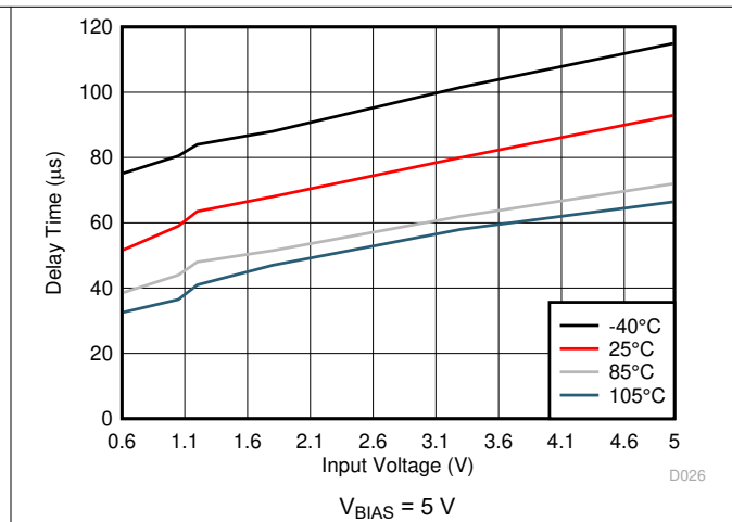
图 6-40. Delay Time vs Input Voltage
