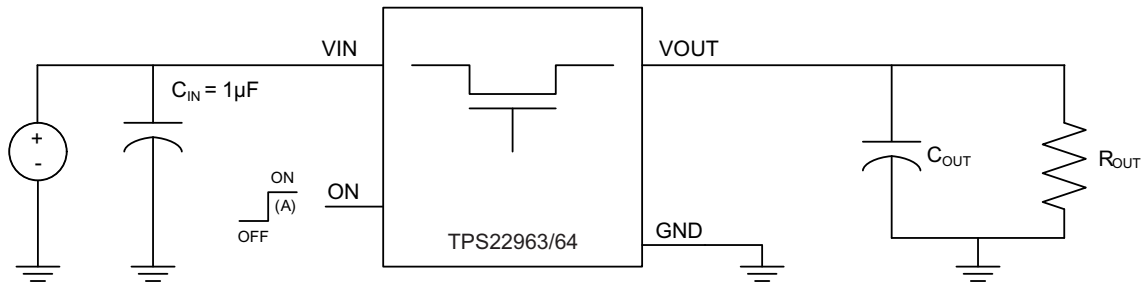
图 36. Test Circuit
