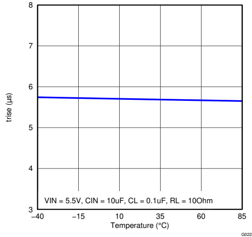
图 5-9. t_R vs Temperature ( V_{IN} = 5.5 V)
