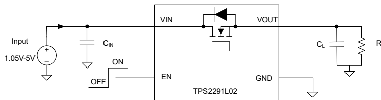
简化版原理图
