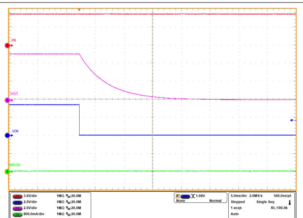
图 8-4. V_{IN} = 5V 且 C_L = 22 \mu F 时 TPS2291L02 的典型关断特性
