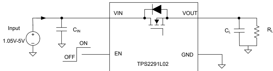
图 8-2. 典型应用图
