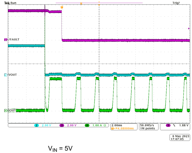
图 8-7. TPS2001E 空载至输出短路
