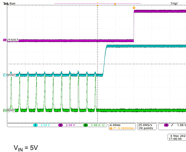
图 8-8. TPS2001E 输出至空载短路
