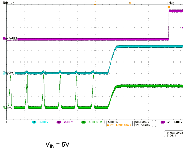
图 8-6. TPS2001E 输出对满载短路
