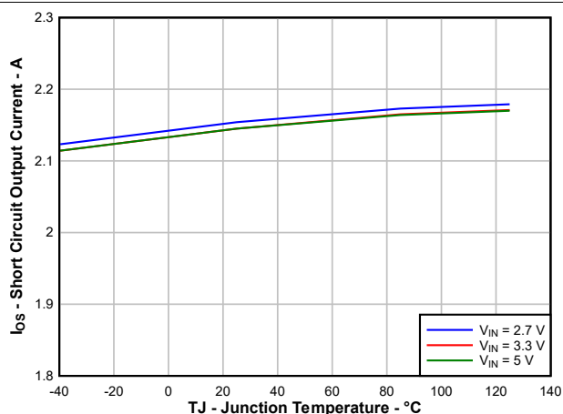
图 6-9. TPS2068E、TPS2069E 短路电流 (I OS ) 与温度间的关系
