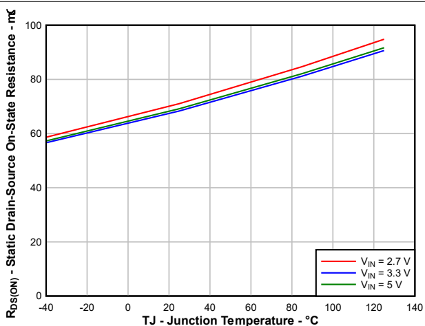
图 6-16. 输入输出电阻 ( R_{DS(ON)} ) 与温度间的关系
