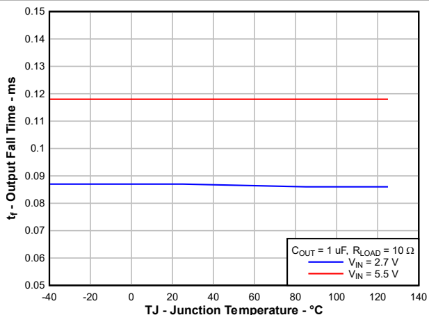
图 6-14. 输出下降时间 ( T_F ) 与温度间的关系
