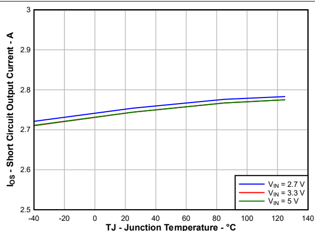
图 6-10. TPS2000E、TPS2001E 短路电流 (I OS ) 与温度间的关系
