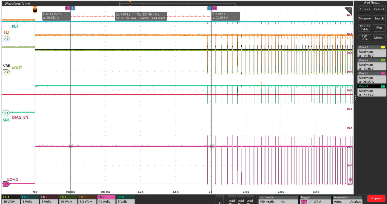
图 8-18. 对于负载电流 (20A 电子负载) 小于电流限制 ( I_{LIM} = GND ) 的情况, 器件进入无限热关断重试阶段
