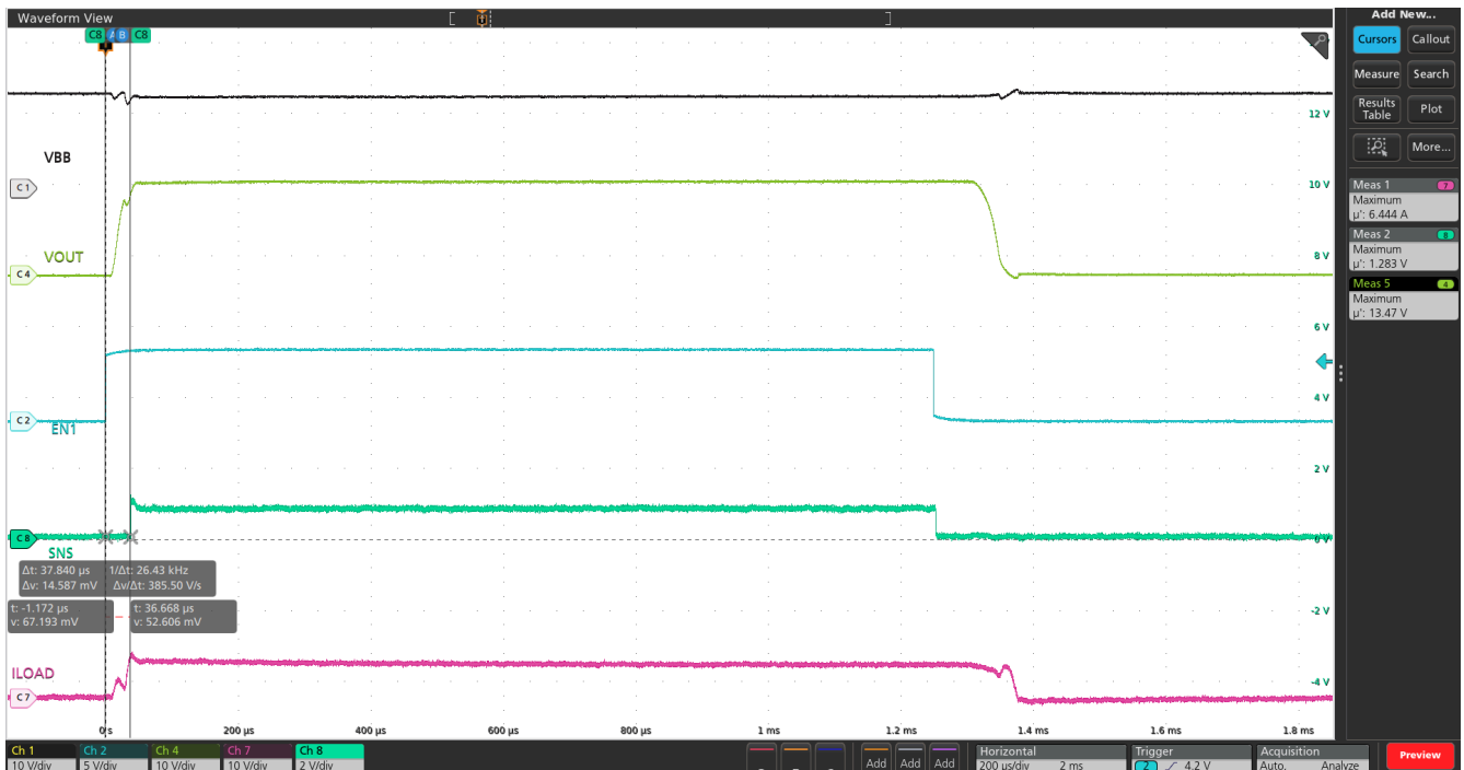
图 8-6. EN 触发的 SNS 响应时间 ( t_{\text{SNSION3}} )
