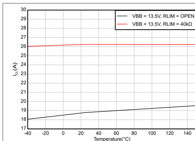
图 6-19. 电流限制调节水平( I_{CL} ) 与温度间的关系
