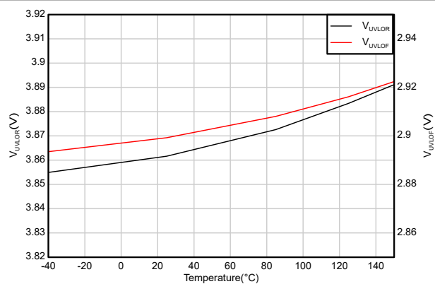
图 6-20. 欠压锁定阈值 ( V_{UVLOR} , V_{UVLOF} ) 与温度间的关系
