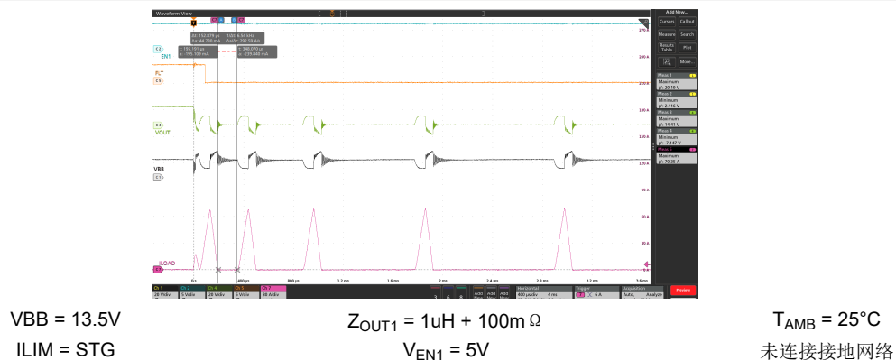
图 9-11. 热短路 (重试行为) 放大至初始重试窗口
