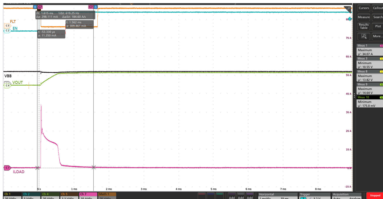
图 8-30. TPS1HC03-Q1 器件在 13.5V VBB、ILIM 引脚开路和 125°C 环境温度下，进行 680uF 容性负载充电
