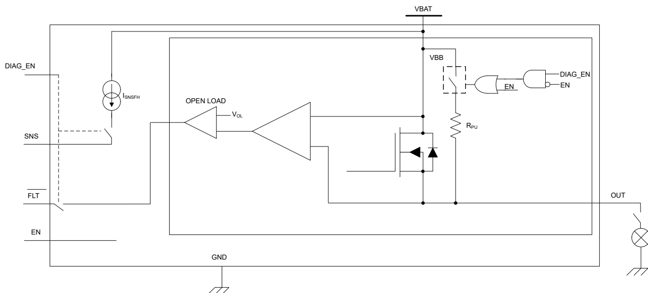
图 8-36. 关断状态下的开路负载检测 ( V_{BB} < V_{DET1} 下降阈值)
