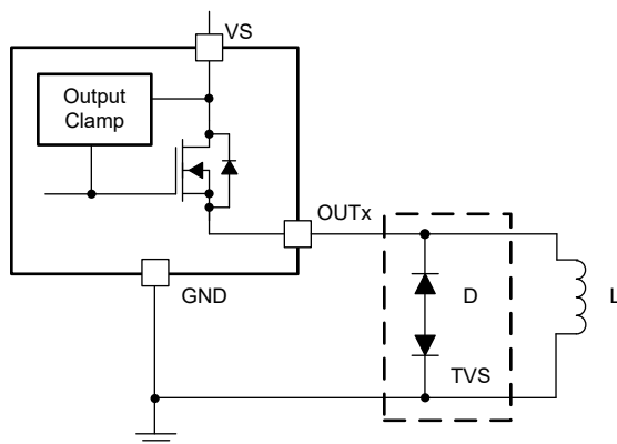
图 8-25. 通过外部电路提供保护
