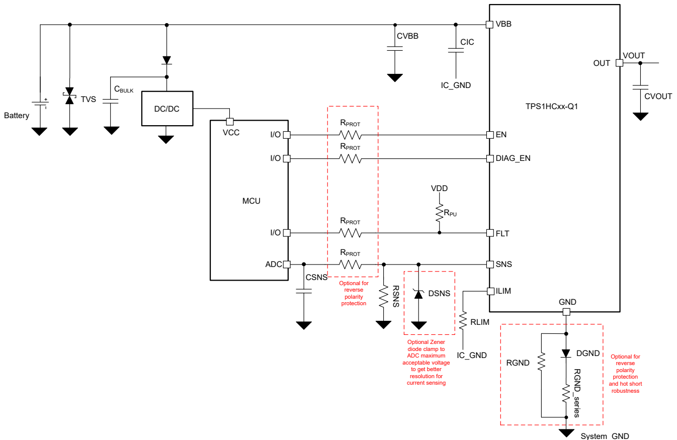
图 9-1. 典型应用图
