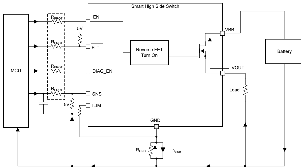
图 8-44. MCU I/O 保护
