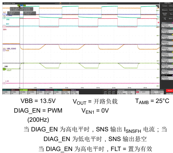
图 9-9. 器件上具有开路负载故障时的开路负载检测延迟 (t OL2 ) (P、D 版本)
