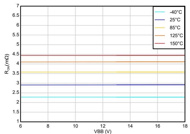
图 6-4. 导通电阻 ( R_{\text{ON}} ) 与 VBB 间的关系
