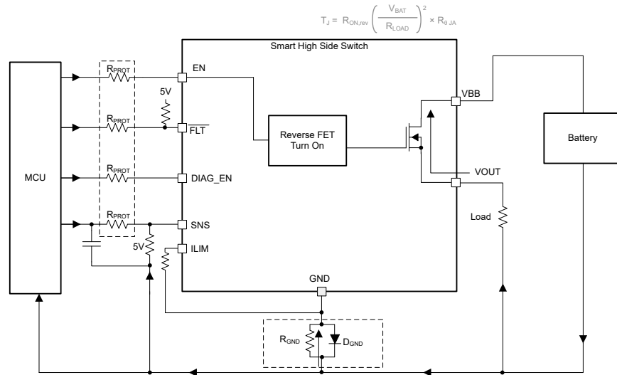
图 8-43. 通过接地网络实现反向保护
