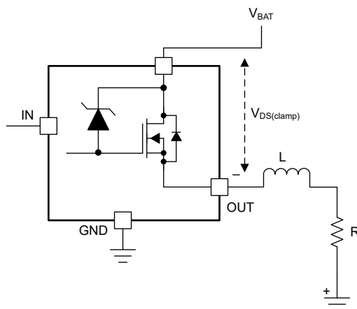
图 8-23. 漏源钳位结构
