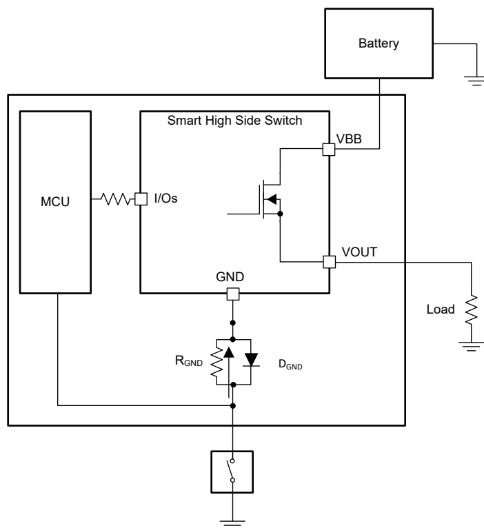
图 8-40. 模块接地失效
