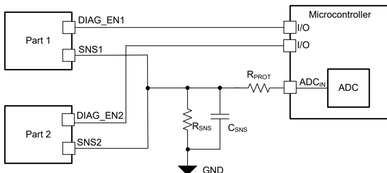
图 8-11. 跨多个器件的 SNS 多路复用
