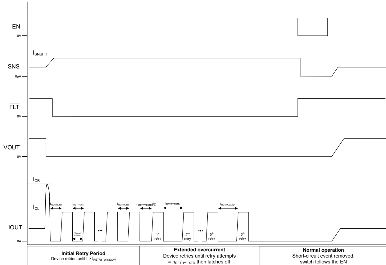
图 8-22. 不使用热调节功能时热短路后的重试行为
