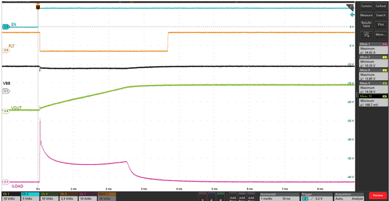
图 8-31. TPS1HC03-Q1 器件在 13.5V VBB、ILIM 引脚开路 and 125°C 环境温度下，进行 2.67mF 容性负载充电
