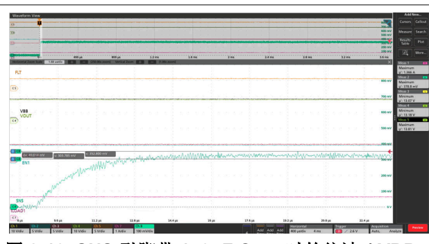
图 8-10. SNS 引脚带 150pF C_{SNS} 时的纹波 ( V_{BB} = 13.5V , I_{LIM} = OPEN , R_L = 10\Omega , R_{SNS} = 1k\Omega , T_A = 25^\circ C )
