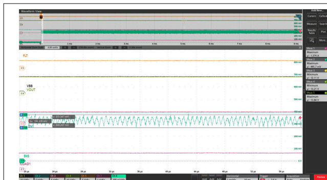
图 8-9. SNS 引脚无 C_{SNS} 时的纹波 ( V_{BB} = 13.5V , I_{LIM} = OPEN , R_L = 10\Omega , R_{SNS} = 1k\Omega , T_A = 25^\circ C )
