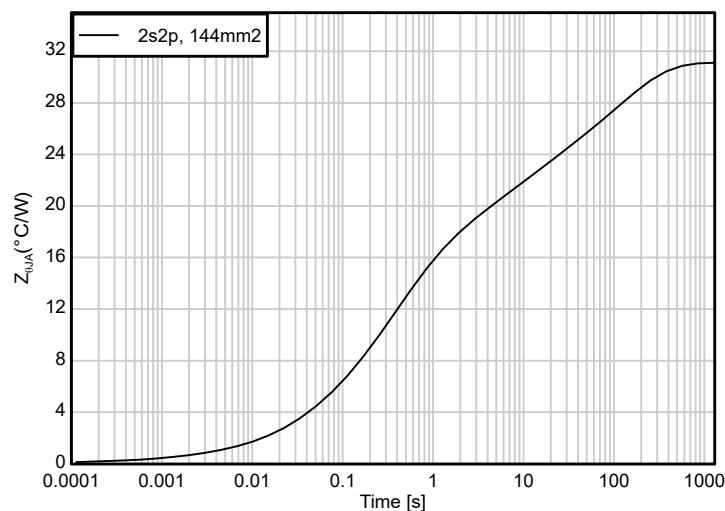
图 9-2. Z_{OJA} (瞬态热阻抗) : JEDEC 标准 2s2p PCB 布局、VBB 和 VOUT 焊盘下方有 5 个过孔
