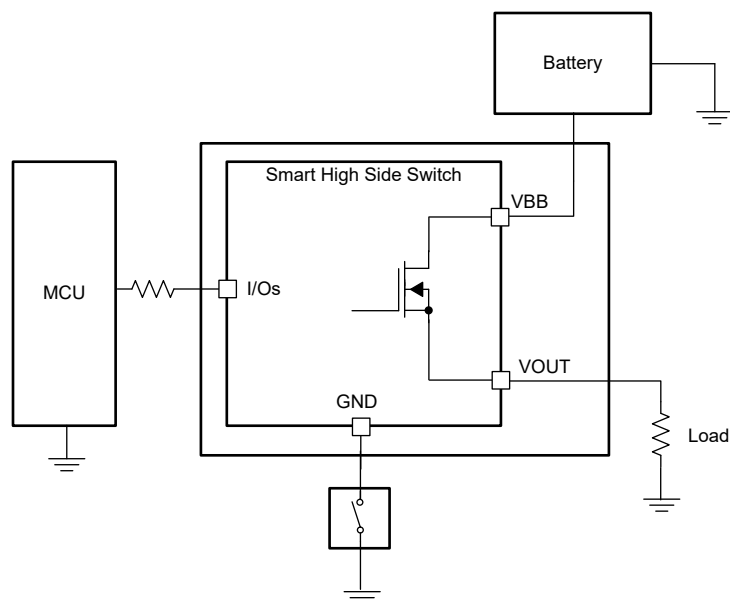
图 8-39. 器件接地失效
