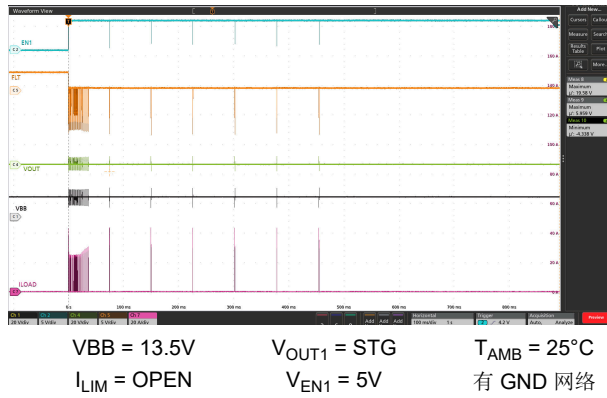
图 9-7. 输出短接至 GND 时的器件导通行为 (ILIM = OPEN)
