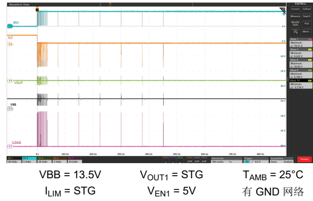
图 9-8. 输出短接至 GND 时的器件导通行为 (ILIM = STG)
