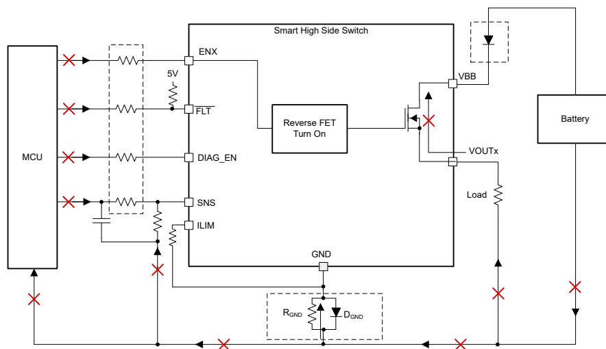
图 8-42. 采用阻断二极管实现反向保护
