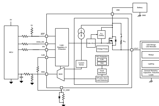
典型应用原理图
