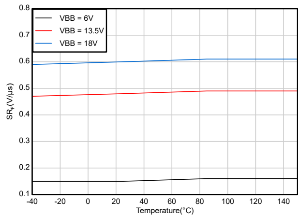
图 6-10. VOUT 下降压摆率 ( SR_F ) 与温度间的关系 (P 版本)
