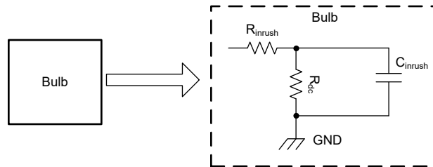
图 8-32. 简单灯泡模型
