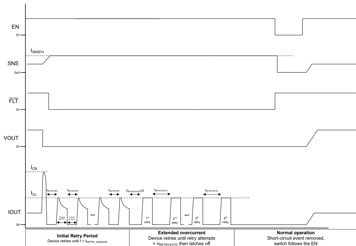
图 8-21. 使用热调节功能时热短路后的重试行为
