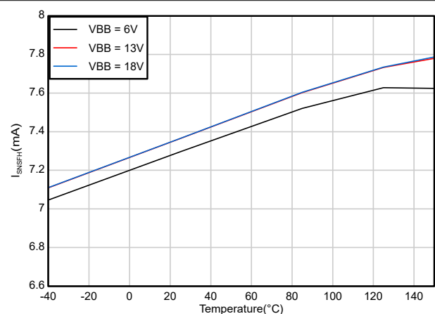
图 6-6. I_{\text{SNS}} 故障高电平电流与温度间的关系
