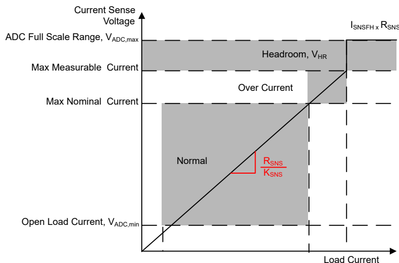
图 8-3. 电流检测引脚上的电压指示
