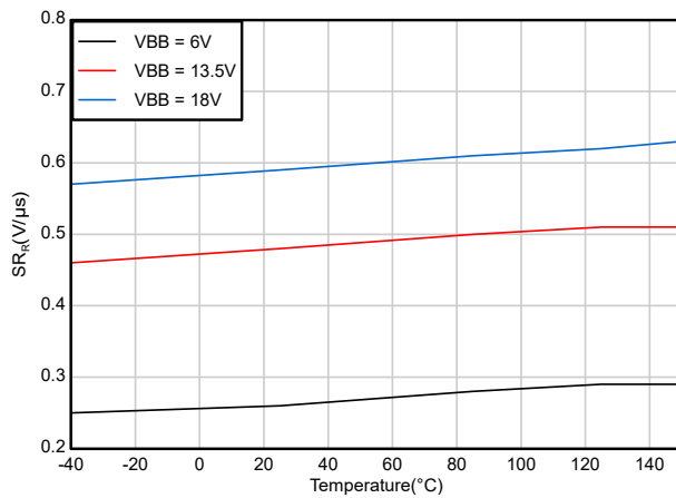
图 6-9. VOUT 上升压摆率 ( SR_R ) 与温度间的关系 (P 版本)
