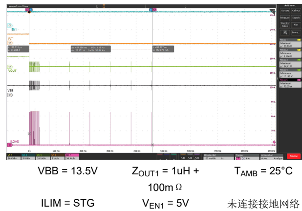
图 9-10. 热短路 (重试行为)
