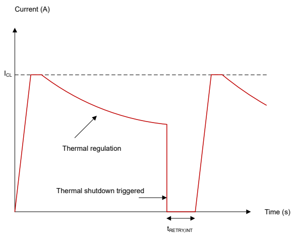
图 8-13. 通过热调节功能使其短路
