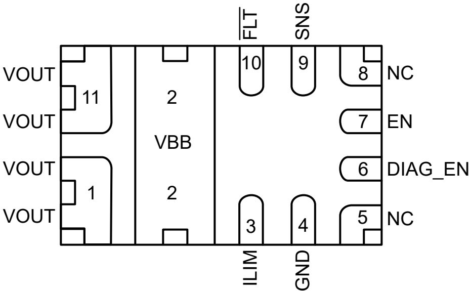
图 5-1. VAH 封装 TPS1HC03-Q1 顶视图
