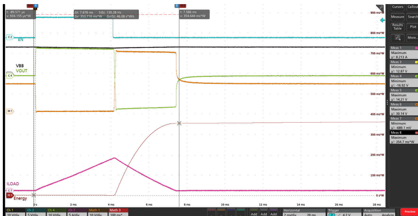
图 8-26. 5mH 电感负载驱动 ( V_{BB} = 13.5V , T_{AMB} = 125^{\circ}C )
