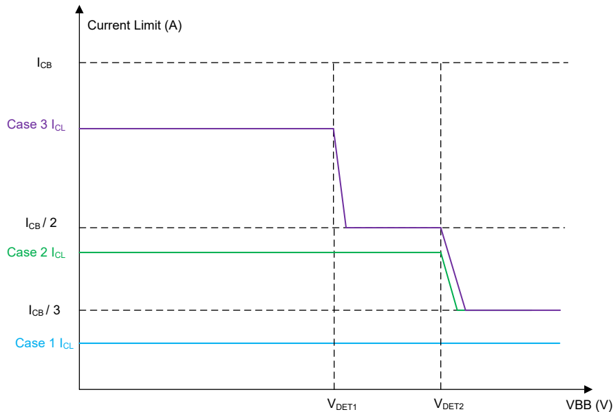
图 8-18. 具有 V_{BB} 的电流限制折返
