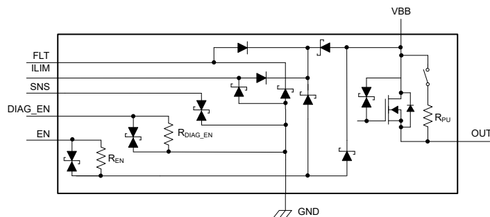
图 8-2. 内部二极管图
