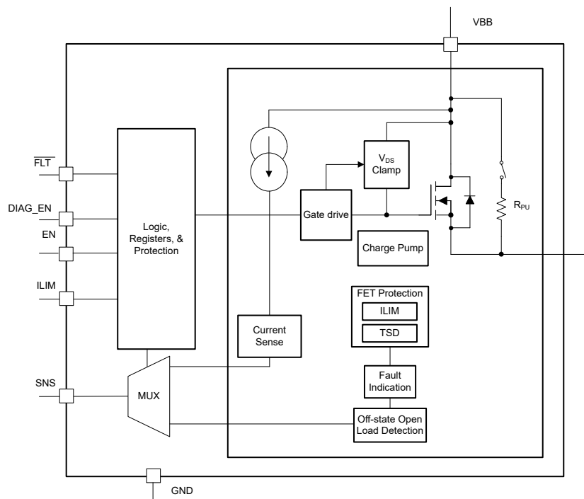
图 8-1. 功能方框图
