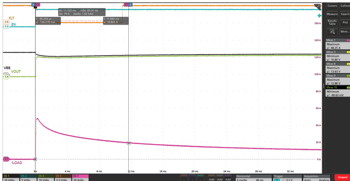
图 8-34. 使用 TPS1HC03-Q1 单通道在 13.5V VBB 下进行 65W 灯泡充电 ( T_A(\text{device}) = 25^\circ\text{C} , T_A(\text{bulb}) = -40^\circ\text{C} , \text{ILIM} = \text{GND} )
