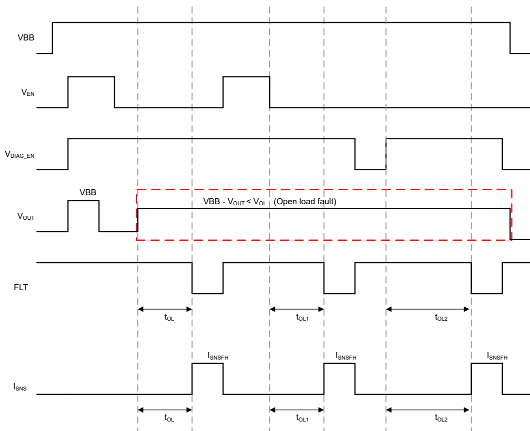
图 8-36. 关断状态下的开路负载检测 ( V_{BB} < V_{DET1} 下降阈值)
