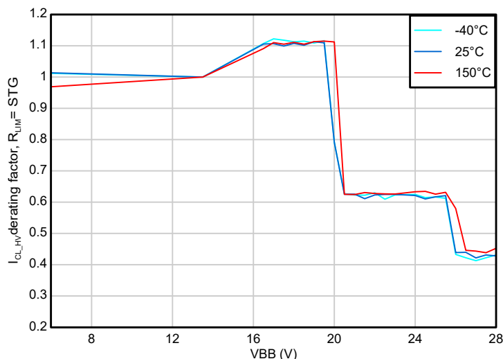
图 8-19. 两个通道的电流限制降额因子 ( I_{CL\_HV} ) 与 VBB 间的关系, R_{LIM} = GND
