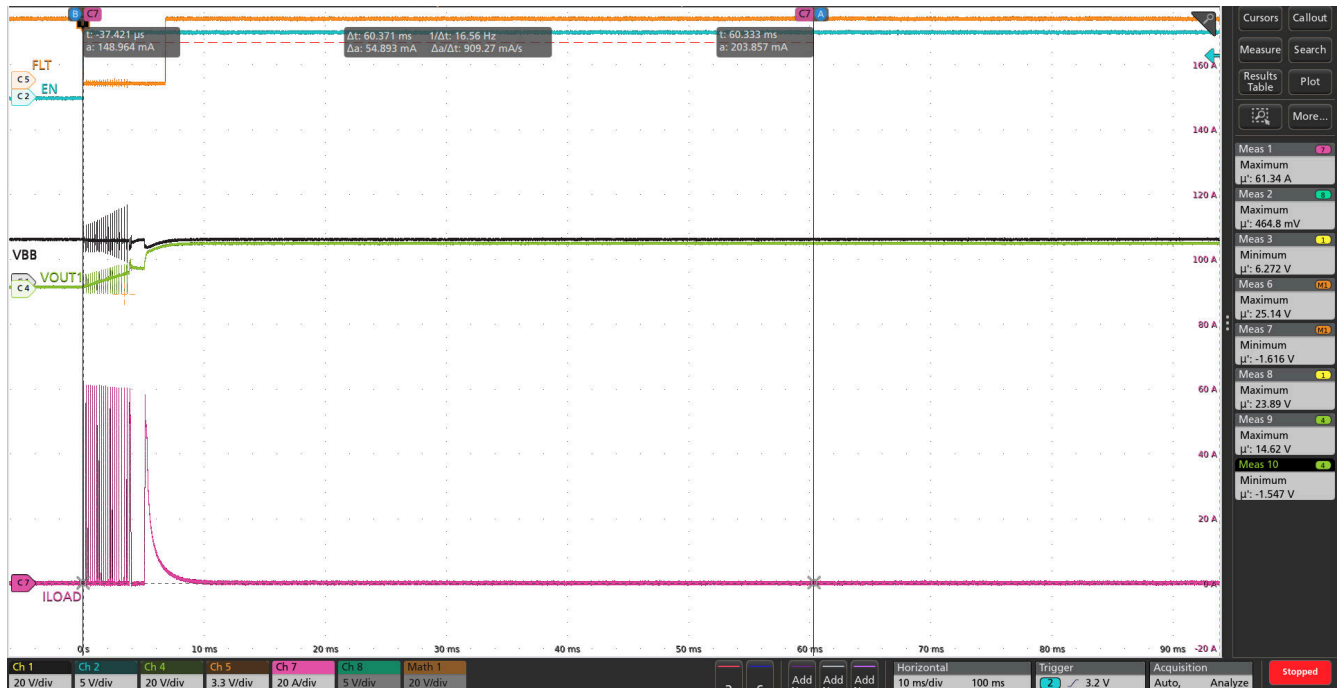
图 8-29. TPS1HC03-Q1 器件在 13.5V VBB、ILIM 引脚短接至地和 125°C 环境温度下，进行 680uF 容性负载充电
