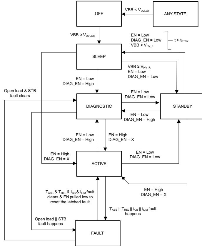
图 8-45. 状态图
