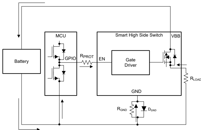
图 8-38. 电池反向电路
