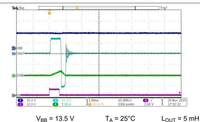
图 7-28. 5-mH Inductive Load Demagnetization
