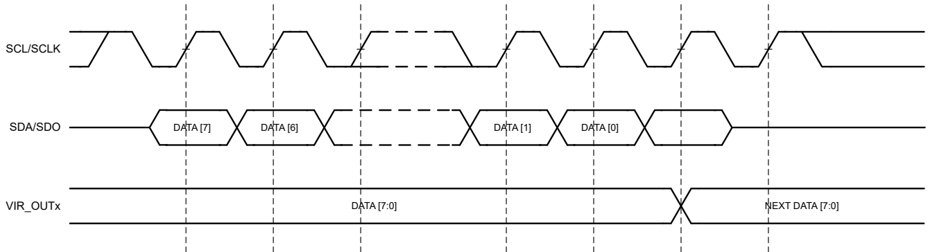
图 7-64. 并行到串行时序的串行通信示例
