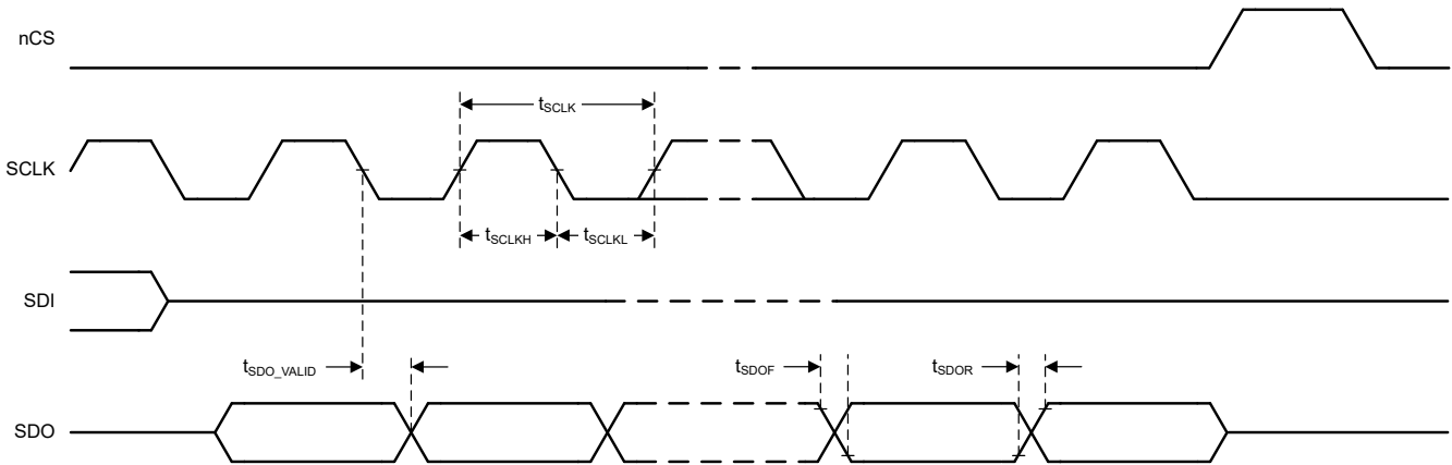
图 7-58. SPI 读取时序图
