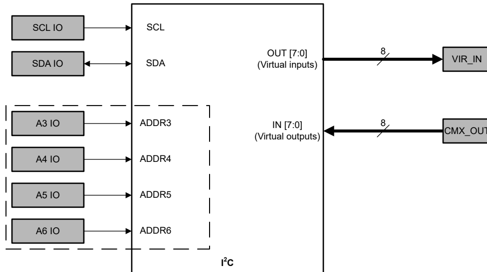
图 7-50. I 2 C 串行通信 GPIO 分配
