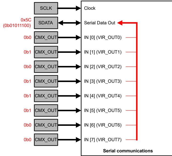
图 7-63. 并行到串行的串行通信方框图
