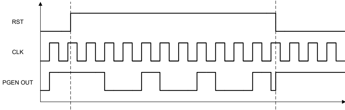
图 7-5. 图形发生器输出时序图示例 ( SIZE = 3 , PATTERN = 100 , 低电平 RST )
