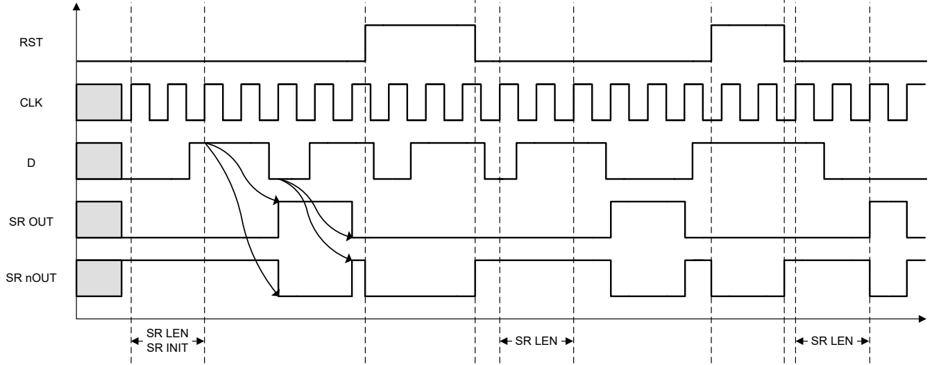
图 7-8. 移位寄存器输出时序图示例 ( INIT 状态 = 00 , REG 长度 = 2 , 高电平 RST )
