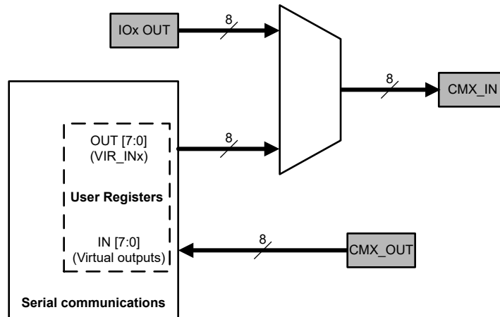
图 7-60. 串行通信方框图
