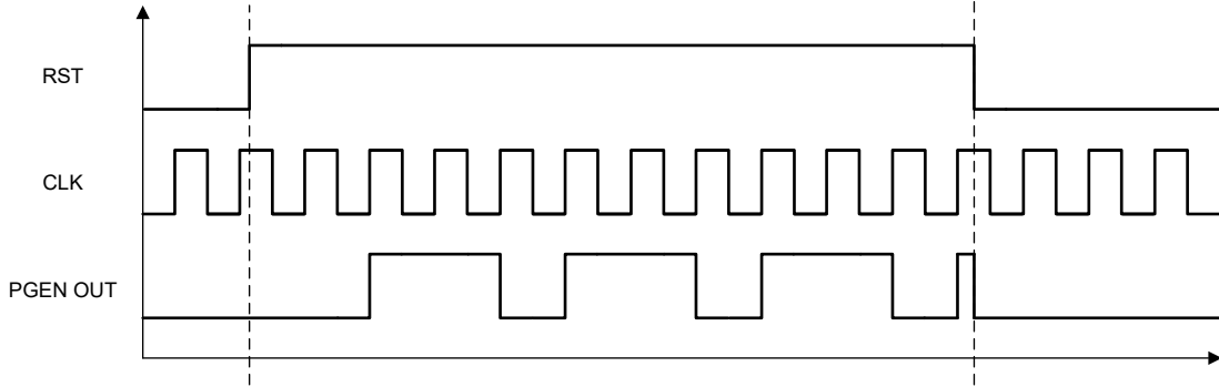
图 7-4. 图形发生器输出时序图示例 ( SIZE = 3 , PATTERN = 011 , 低电平 RST )
