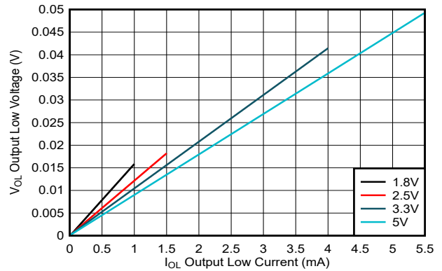
图 6-4. 低电平状态下的典型 2X 推挽输出电压 ( V_{OL} )
