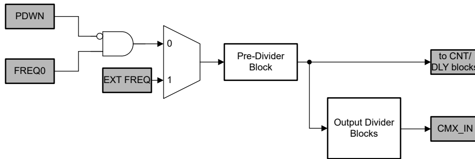
图 8-48. 固定频率振荡器方框图
