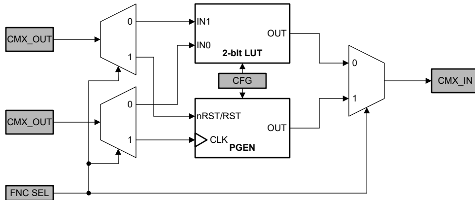
图 8-3. 2 位 LUT 或图形发生器方框图
