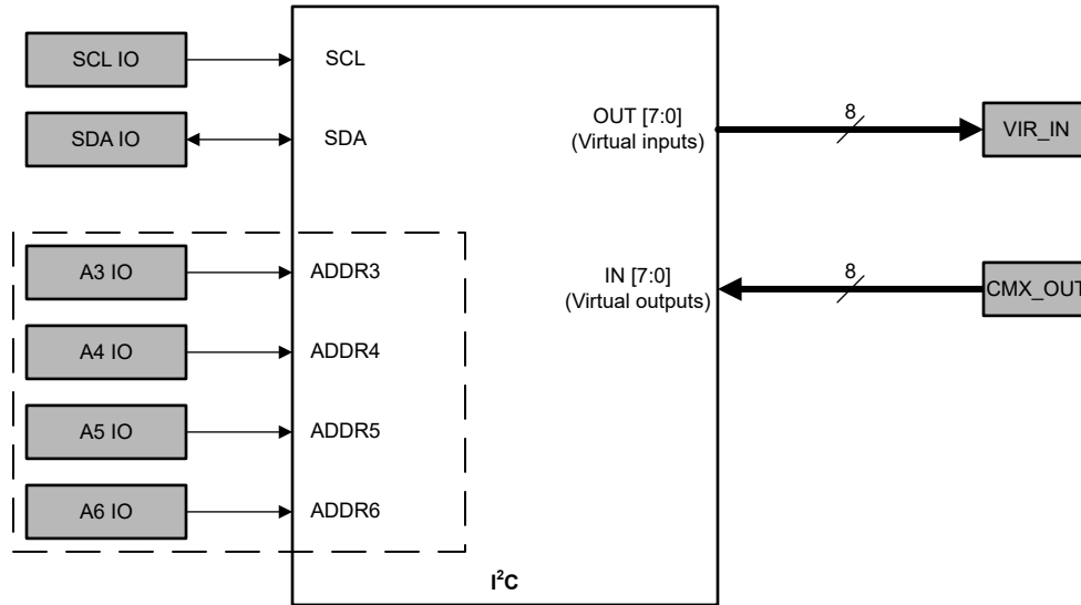
图 8-50. I 2 C 串行通信 GPIO 分配
