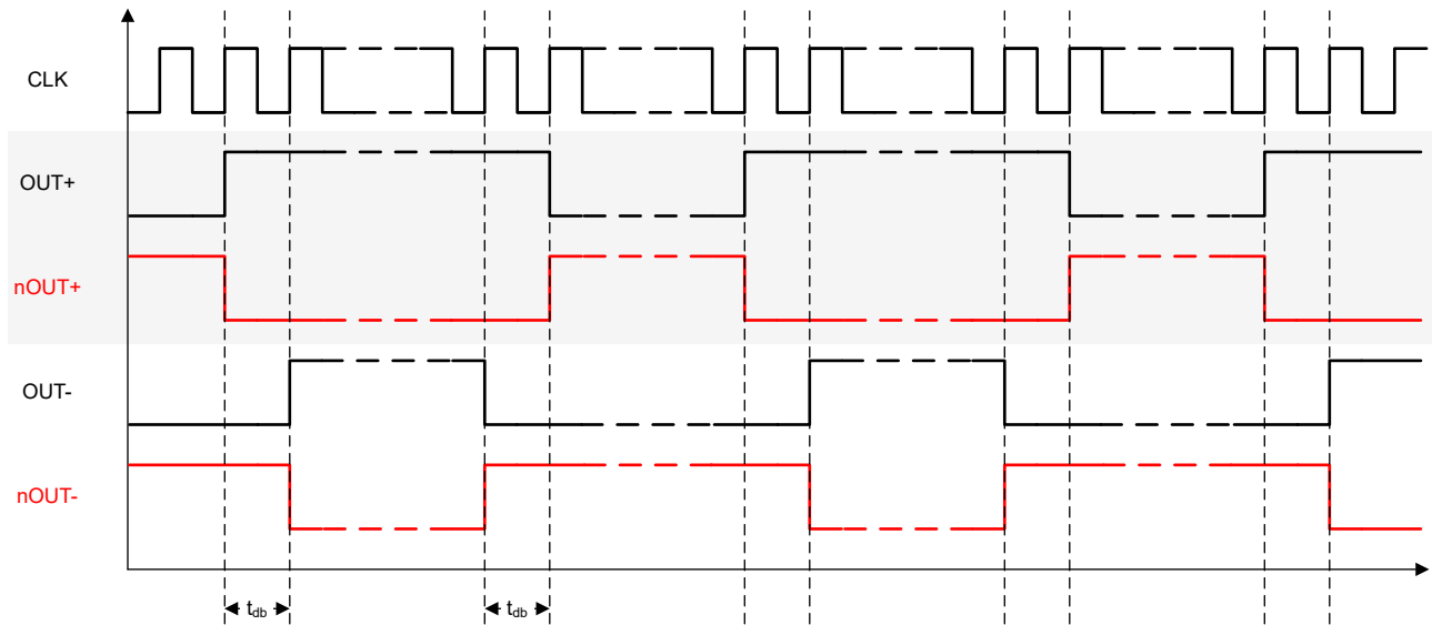
图 8-39. PWM 发生器时序示例
