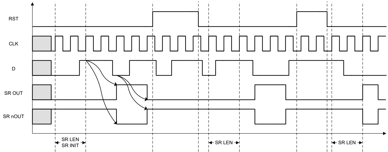
图 8-8. 移位寄存器输出计时示意图示例 ( 初始状态 = 00 , 寄存器长度 = 2 , 高电平 RST )
