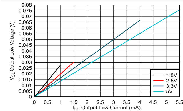
图 6-5. 低电平状态下的典型 1X 开漏 NMOS 输出电压 ( V_{OL} )
