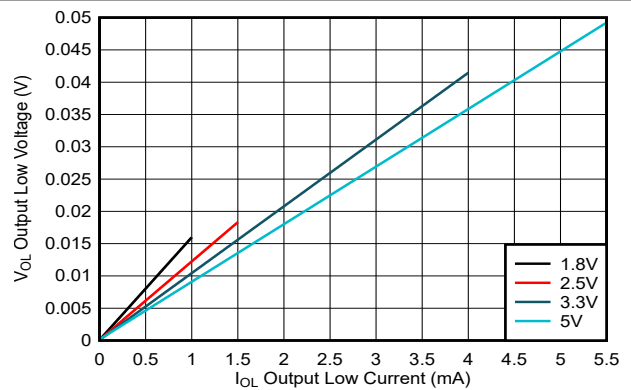
图 6-6. 低电平状态下的典型 2X 开漏 NMOS 输出电压 ( V_{OL} )
