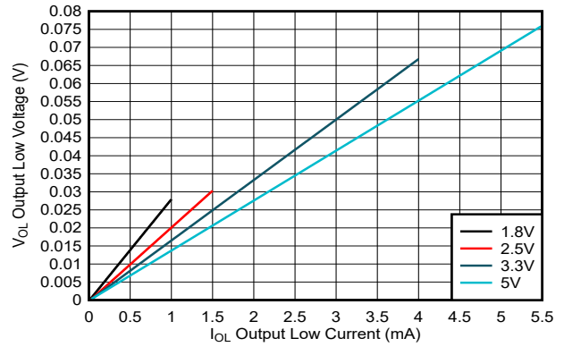
图 6-2. 低电平状态下的典型 1X 推挽输出电压 ( V_{OL} )
