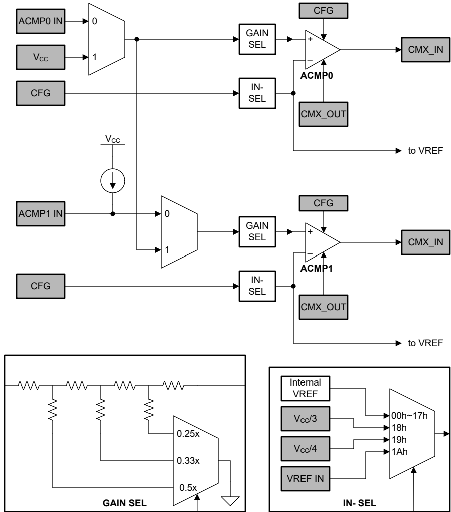
图 7-20. ACMP 方框图
