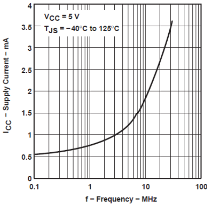
图 5-1. 电源电流与频率间的关系
