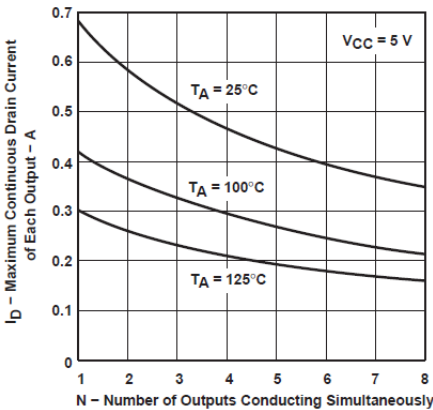
图 5-2. 每个输出的最大连续漏极电流与同时导通的输出数量之间的关系
