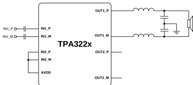
图 44. Mono BTL
