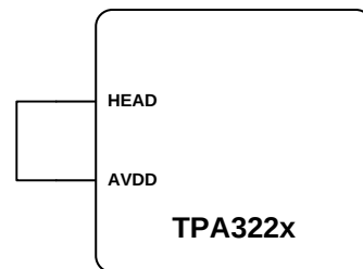
图 35. HEAD-Mode Configuration
