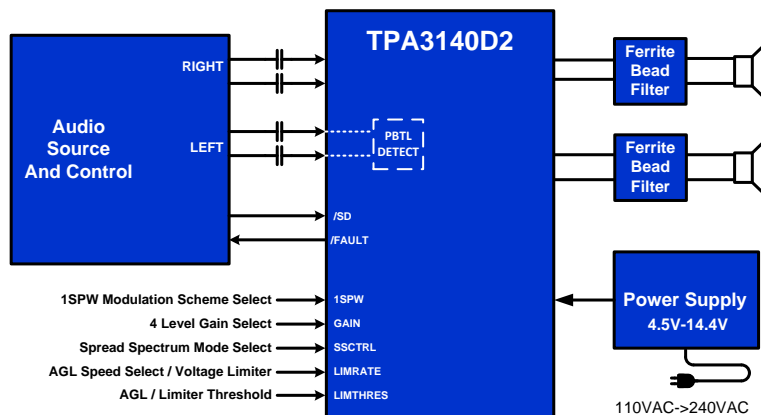
简化原理图
