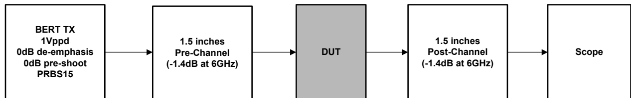
图 8-3. 测试设置
