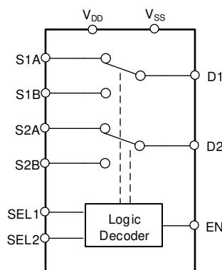
方框图
