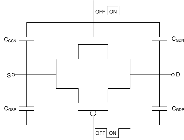
图 8-12. 传输门拓扑
