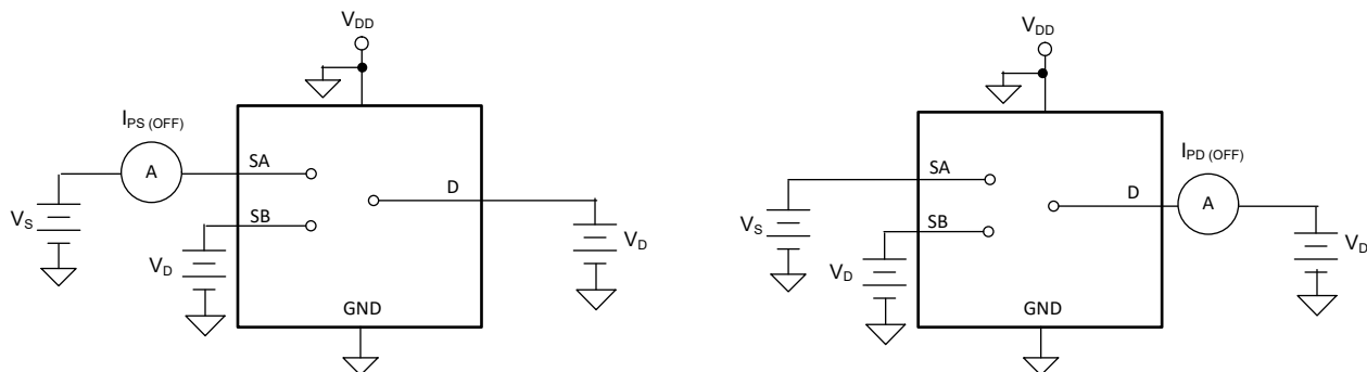
图 6-4. 断电漏电流测量设置
