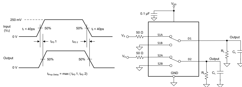
图 6-12. 带宽测量设置
