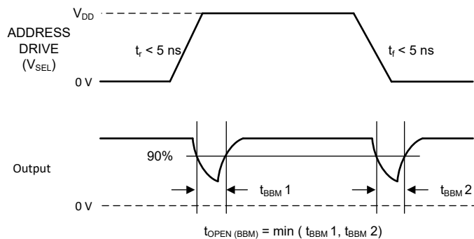
图 6-8. 先断后合延迟测量设置
