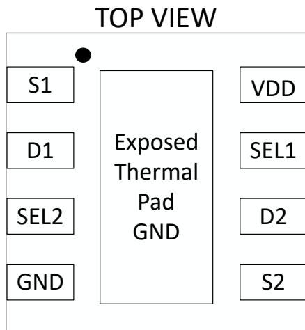
图 4-1. DSG 封装 TMUX2821 ( 1:1 双通道 )
