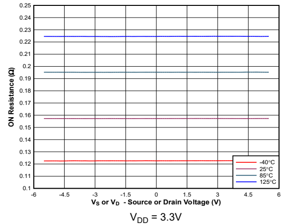
图 5-2. 不同温度下导通电阻与源极或漏极电压间的关系
