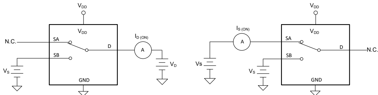
图 6-2. 导通漏电流测量设置
