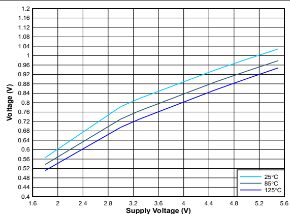
图 5-8. V_{IL} 逻辑阈值与电源电压间的关系
