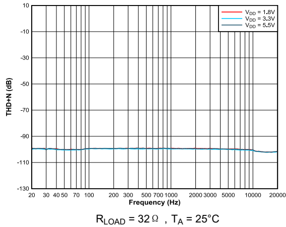
图 5-13. THD+N 与频率间的关系
