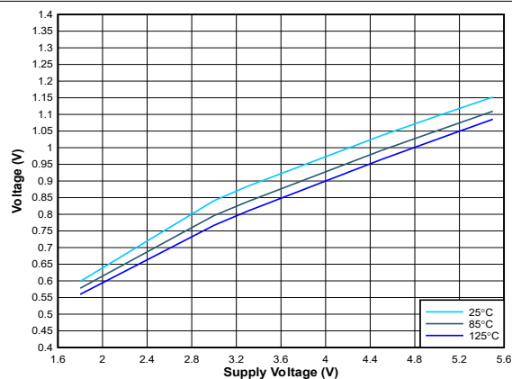
图 5-7. V_{IH} 逻辑阈值与电源电压间的关系
