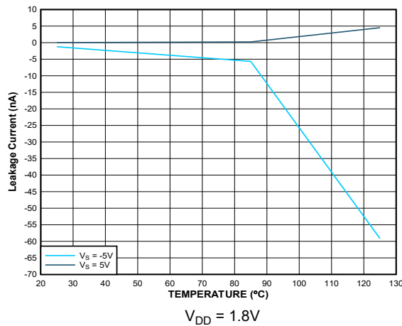
图 5-3. ION 漏电流与温度间的关系
