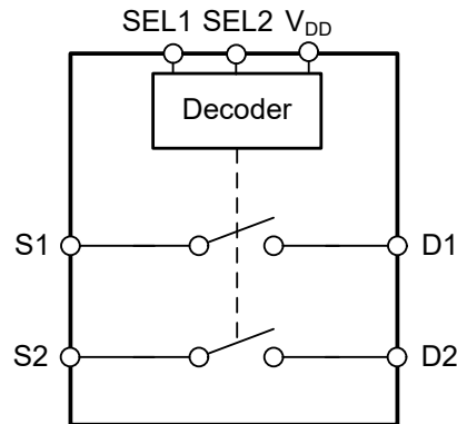
TMUX2819 和 TMUX2821 方框图
