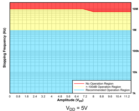
图 5-17. 最大正弦信号摆幅
