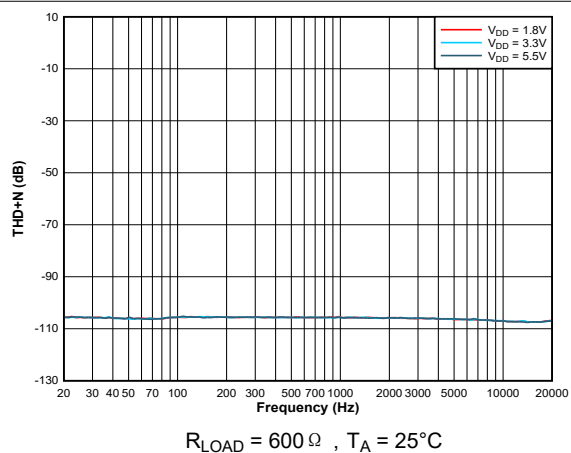
图 5-12. THD+N 与频率间的关系
