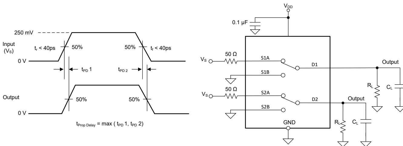
图 6-6. t_{ON}(VDD) 和 t_{OFF}(VDD) 时间测量设置
