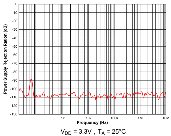
图 5-16. ACPSRR 与频率间的关系
