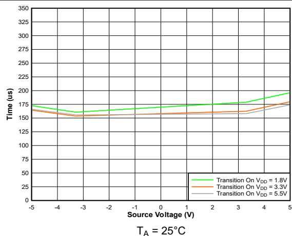
图 5-9. 转换时间与源极电压间的关系
