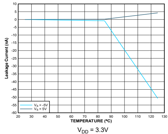
图 5-4. ION 漏电流与温度间的关系
