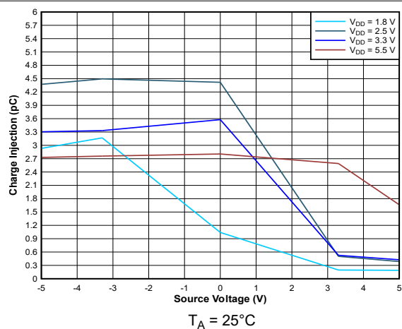
图 5-11. 电荷注入与源极电压间的关系
