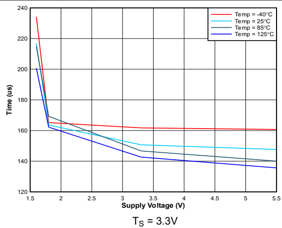
图 5-10. t_{BBM} 与电源电压间的关系
