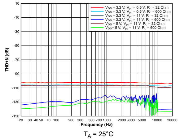
图 5-14. THD+N 与频率间的关系
