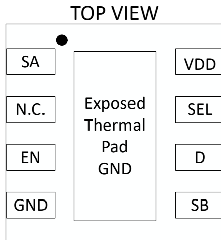
图 4-2. DSG 封装 TMUX2819 ( 2:1 单通道 )
