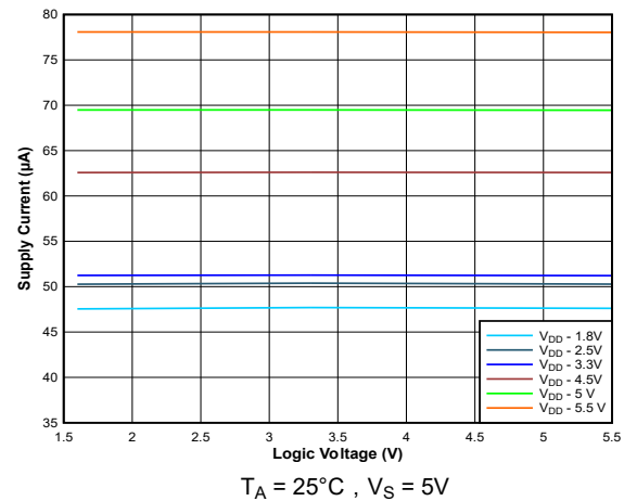
图 5-6. 电源电流与逻辑电压间的关系
