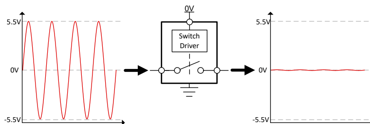
图 7-2. 超出电源电压的断电保护
