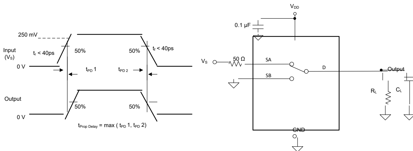
图 6-5. 传播延迟测量设置
