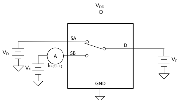
图 6-3. 关断漏电流测量设置
