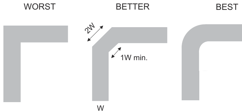
图 8-3. 布线示例
