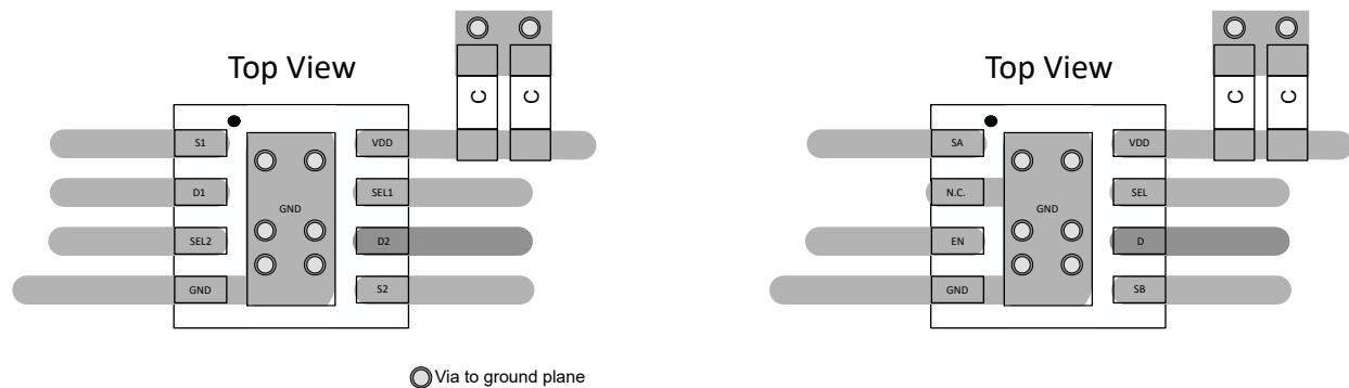
图 8-4. TMUX28xx 布局示例
