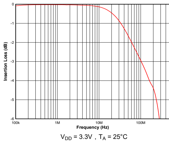
图 5-15. 插入损耗与频率间的关系
