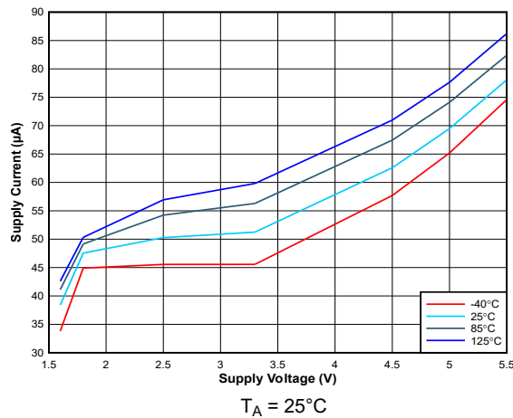
图 5-5. 电源电流与电源电压间的关系
