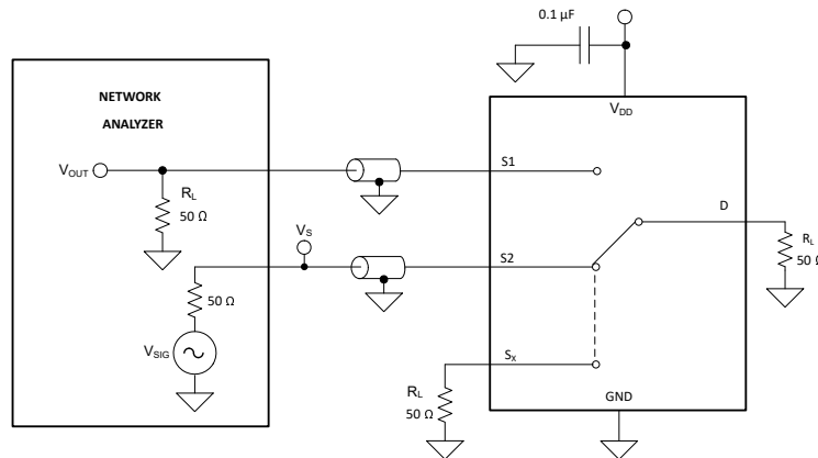
图 6-10. 通道间串扰测量设置
