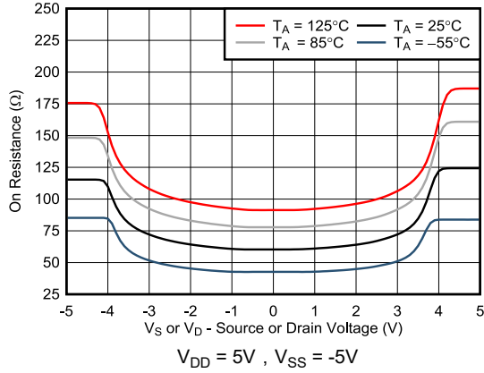
图 5-1. 导通电阻与温度间的关系
