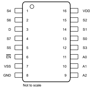
图 4-1. TMUX182-SEP DYY 封装，16 引脚 SOT-23-THIN（顶视图）
