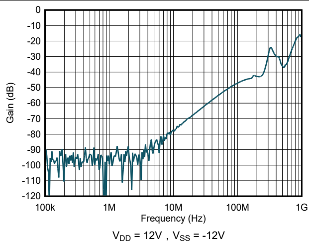
图 5-8. 关断隔离与频率间的关系
