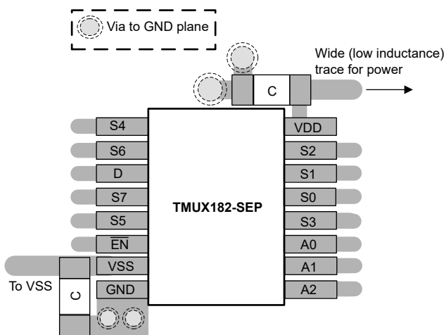
图 8-3. 布局示例
