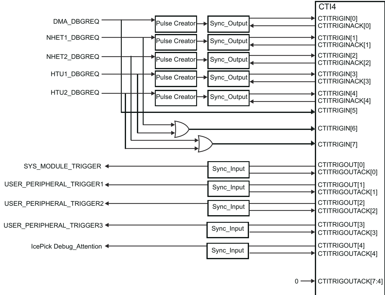
图 7-27. CTI4 Mapping
