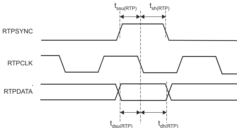
图 7-33. RTPDATA Timing
