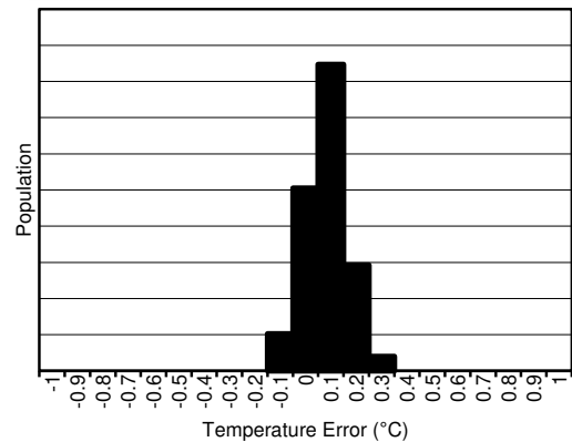
图 6-6. 25 ^\circ\text{C} 时的温度误差
