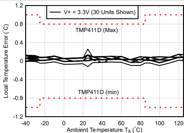
图 9-9. 本地温度误差与 TMP411D 环境温度间的关系
