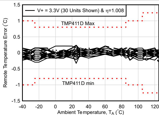
图 9-8. 远程温度误差与 TMP411D 环境温度间的关系
