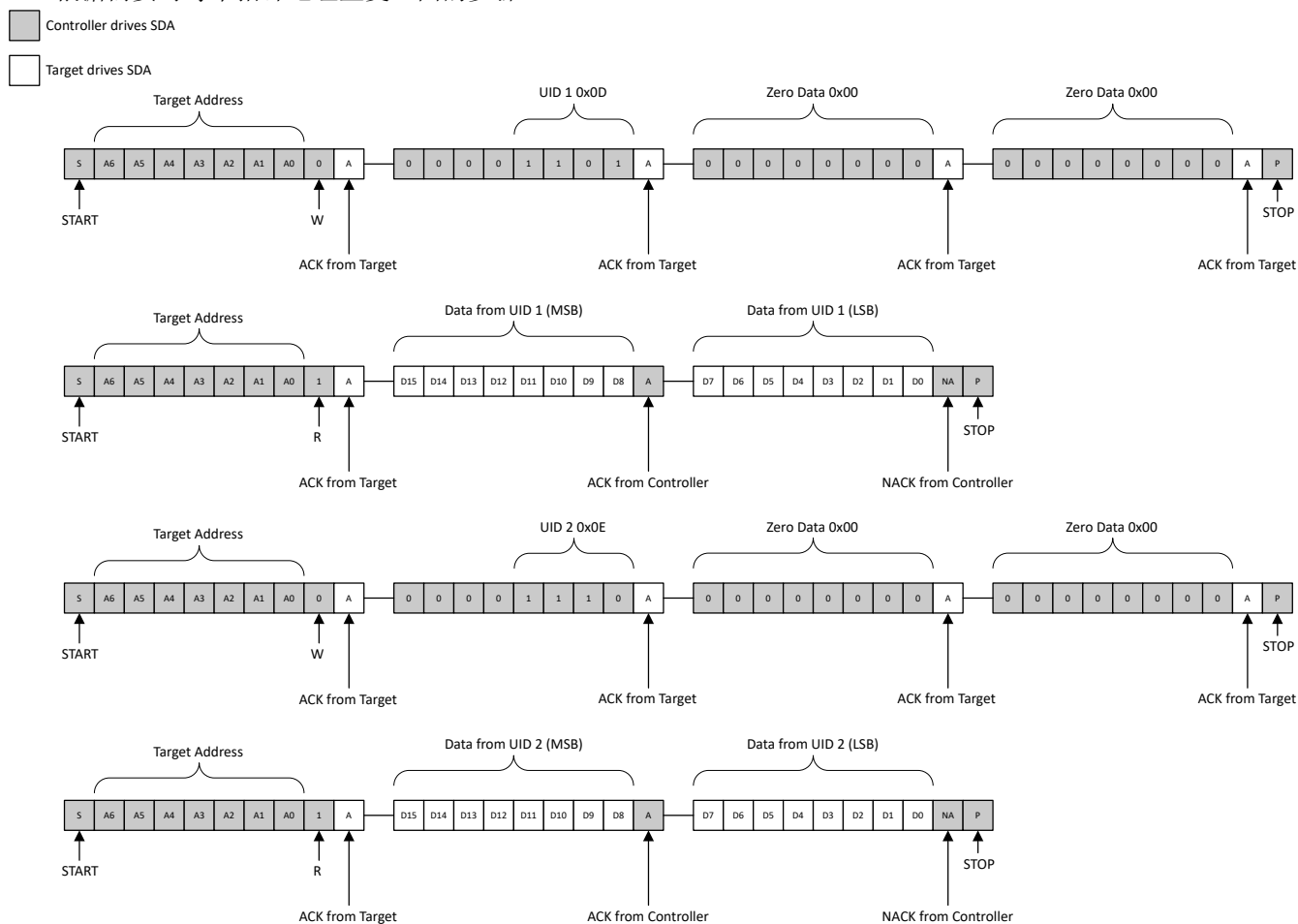
图 7-10. 继续从 UID 1 和 UID 2 读取内容
