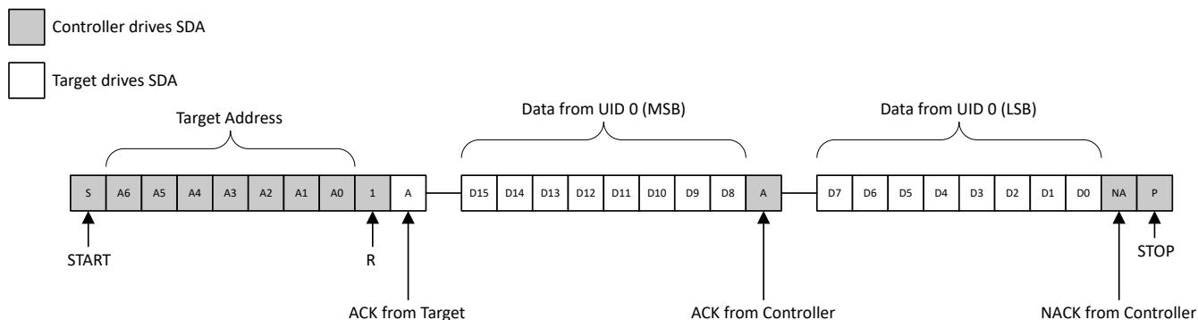
图 7-9. 从 UID 0 读取内容
