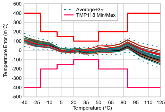
图 6-2. TMP118 温度误差与温度间的关系
