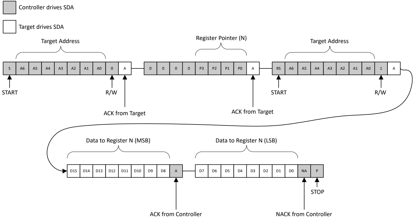
图 7-16. 从单个寄存器读取
