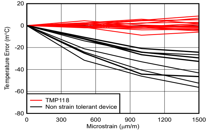
图 7-6. 温度误差与应变间的关系
