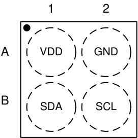
图 5-1. YMS 封装，4 引脚 PICOSTAR ( 顶视图 )
