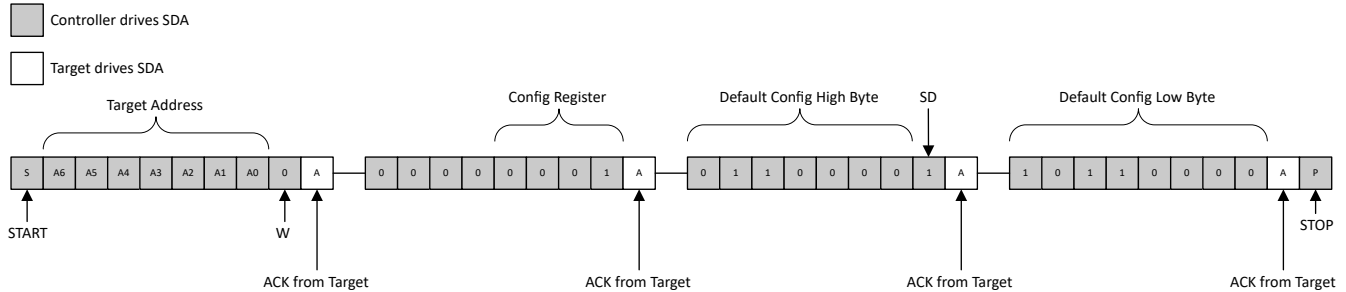
图 7-7. 将器件置于关断 (SD) 模式
