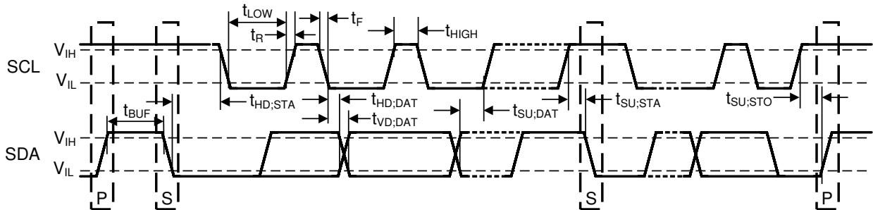
图 6-1. 两线制接口时序图
