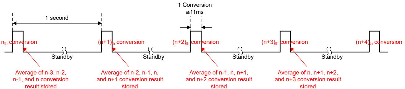
图 7-4. 4 次移动均值计算时的转换情况 (1Hz 转换周期)
