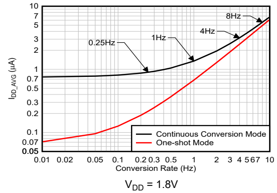
图 6-15. 平均静态电流与转换率间的关系
