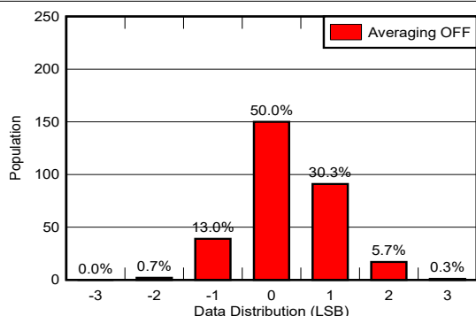
图 6-8. 温度数据噪声分布
