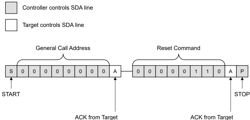
图 7-17. SMBus 通用广播复位图
