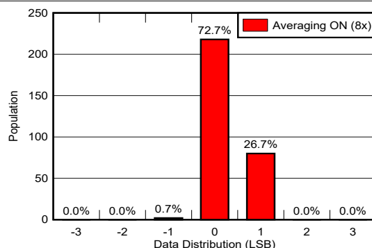
图 6-9. 温度数据噪声分布
