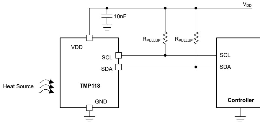
图 9-2. 相同的 I 2 C 上拉和电源电压应用
