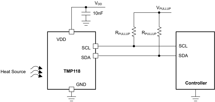
图 9-1. 单独的 I2C 上拉和电源电压应用
