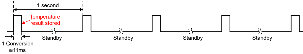
图 7-2. 无均值计算时的转换情况 (1Hz 转换率示例)
