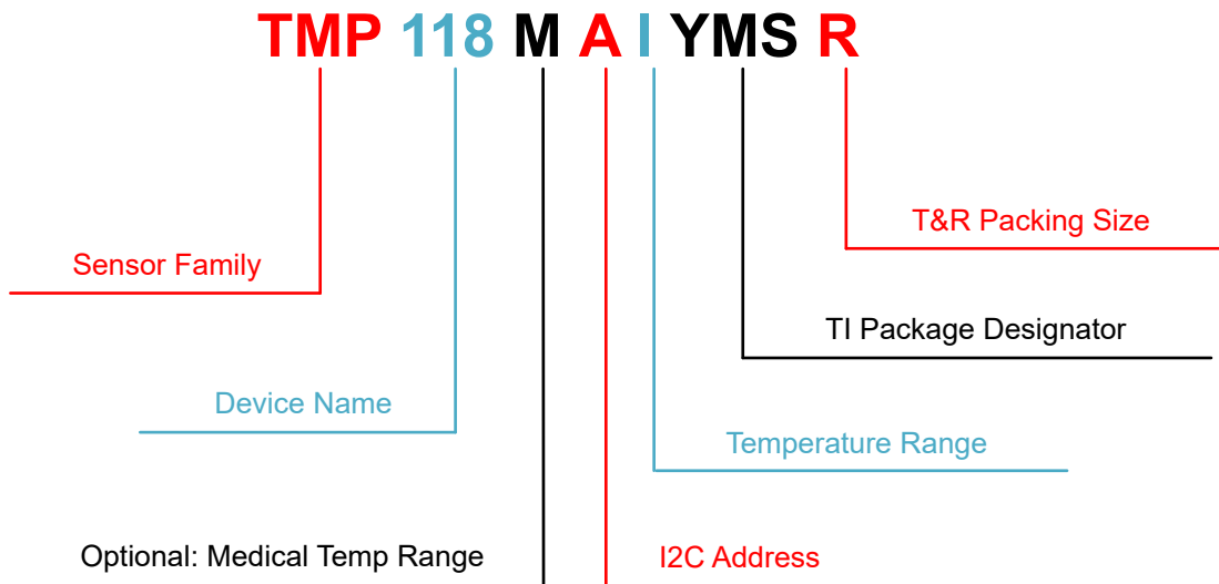
图 4-1. TMP118 器件命名规则
