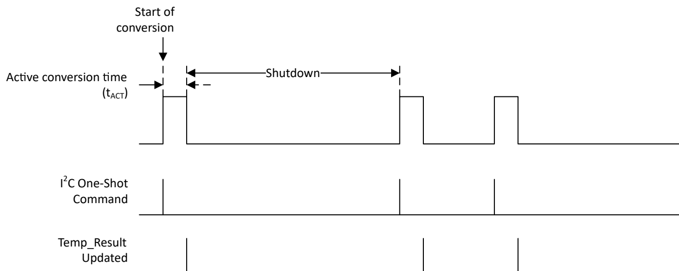
图 7-12. 单稳态时序图
