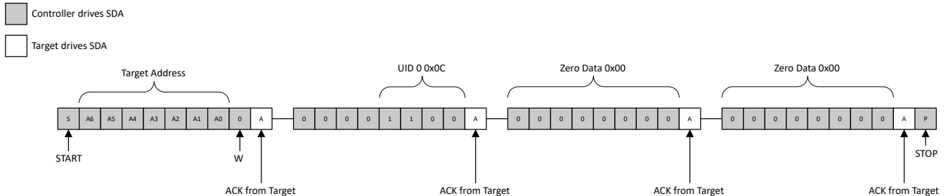
图 7-8. 将 0x0000 写入唯一 ID 0 (UID 0)
