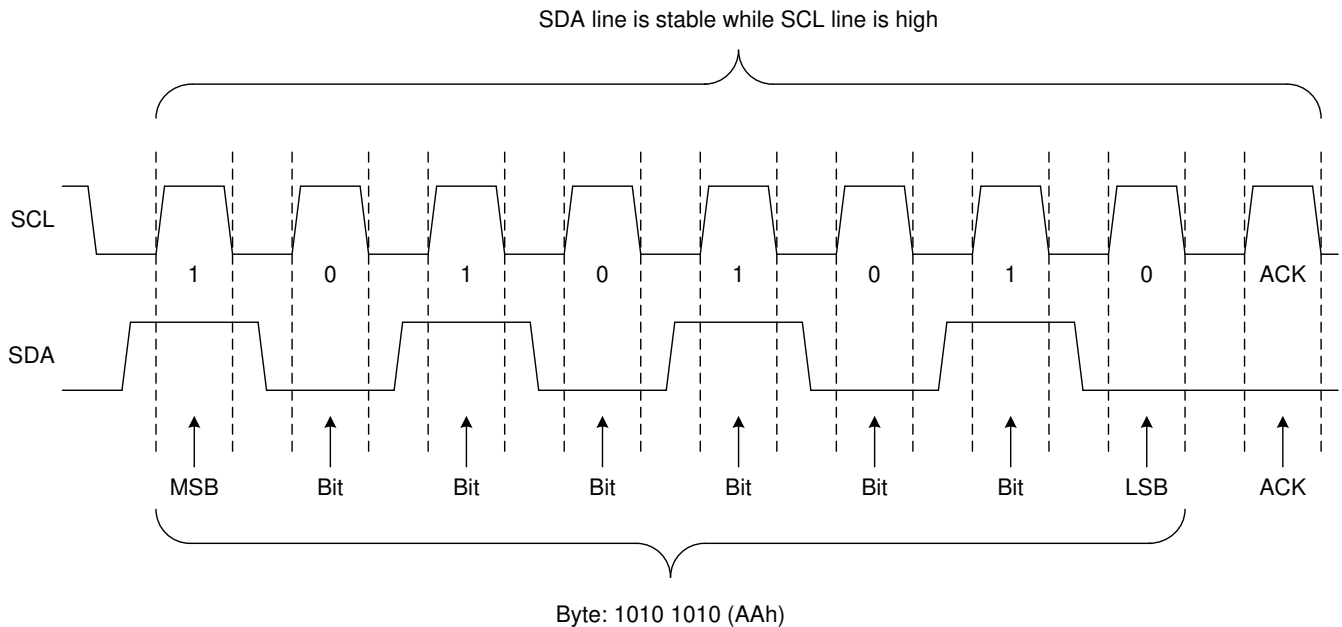
图 7-14. 一个字节的传输
