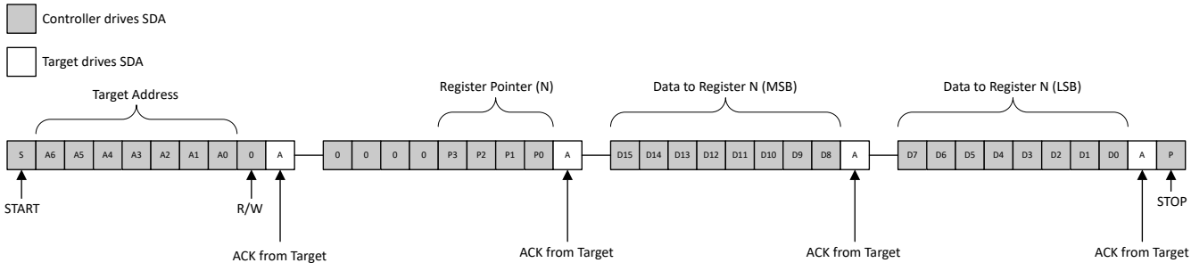
图 7-15. 向单个寄存器写入
