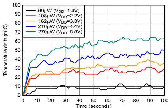
图 6-20. 温度测量响应时间
