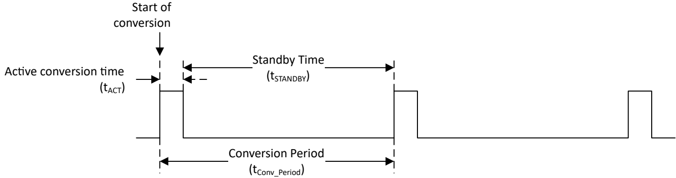
图 7-11. 连续转换周期时序图
