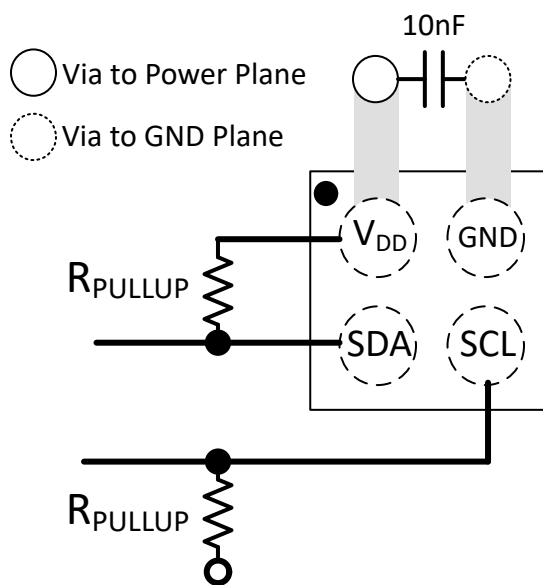
图 9-3. YMS 布局建议
