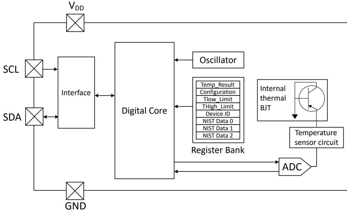
图 7-1. 内部框图
