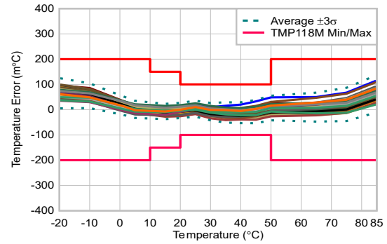
图 6-5. TMP118M 温度误差与温度间的关系
