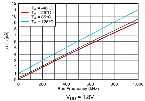
图 6-19. 关断电流与总线频率间的关系
