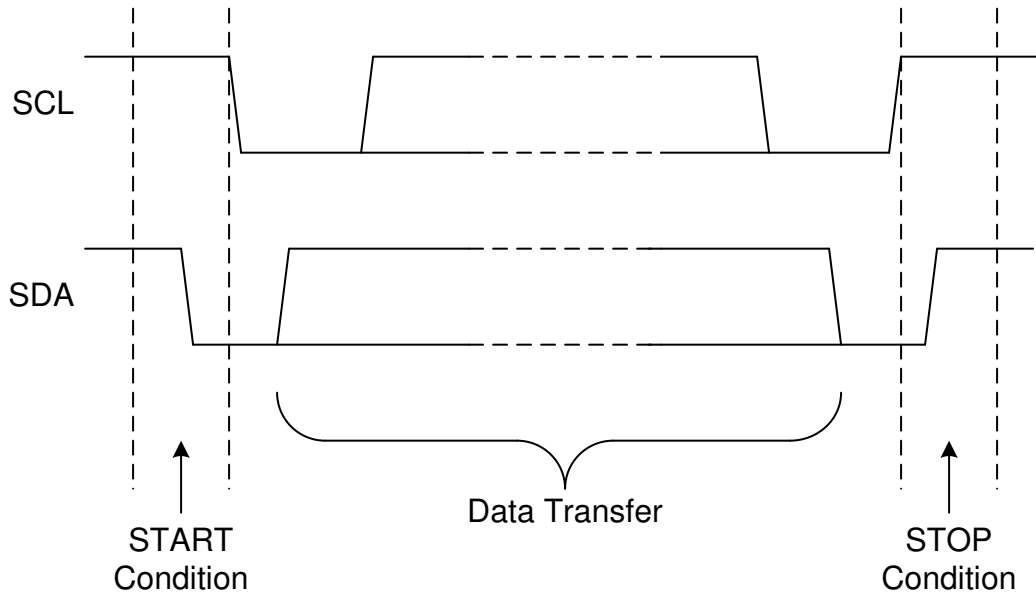
图 7-13. 启动和停止条件的定义
