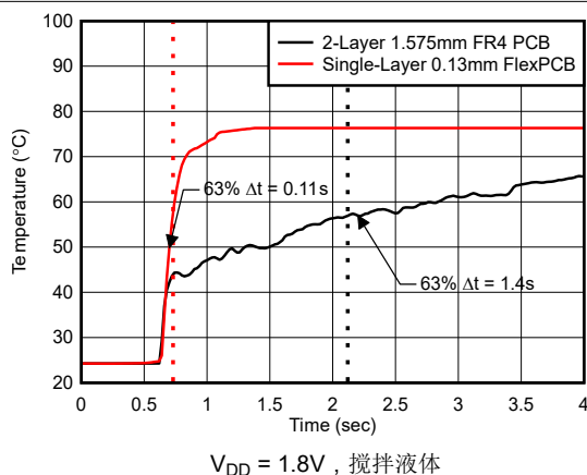
图 6-20. 温度测量响应时间
