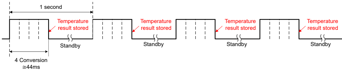
图 7-3. 4 次背靠背均值计算时的转换情况 (1Hz 转换率示例)
