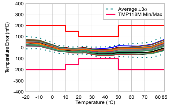
图 6-3. TMP118M 温度误差与温度间的关系
