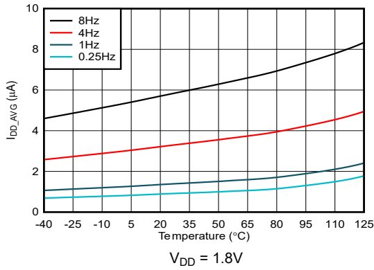
图 6-14. 平均静态电流与温度间的关系
