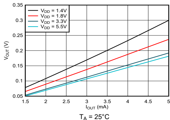
图 6-23. SDA 输出电压与负载电流间的关系
