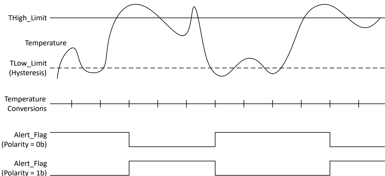
图 7-5. Alert_Flag 行为
