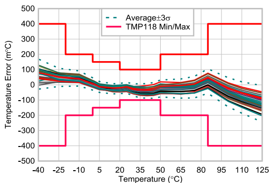
TMP118 温度精度 (1.8V 电源)
