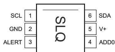
图 5-1. DRL 封装 6 引脚 SOT563 顶视图
