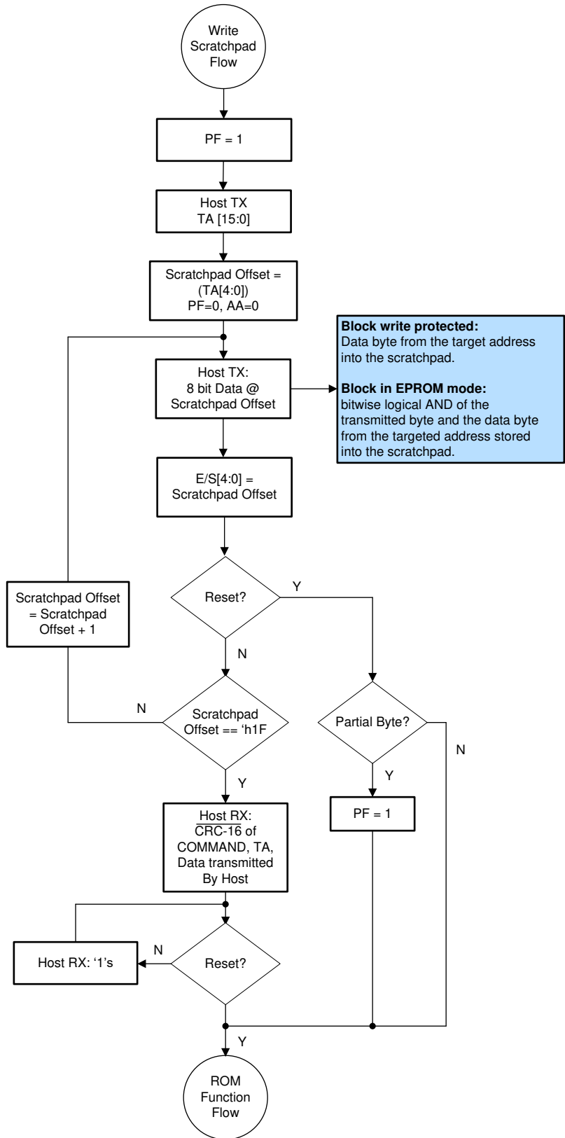
图 6-12. 写入暂存区流程图
