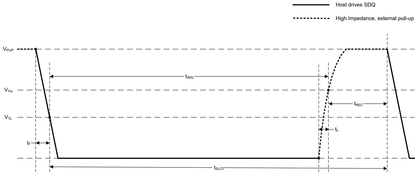
图 6-19. 写入“0”时序图
