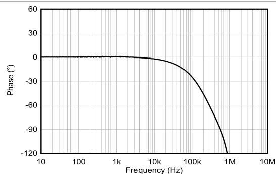
图 6-2. 相位与频率间的关系 (所有增益)
