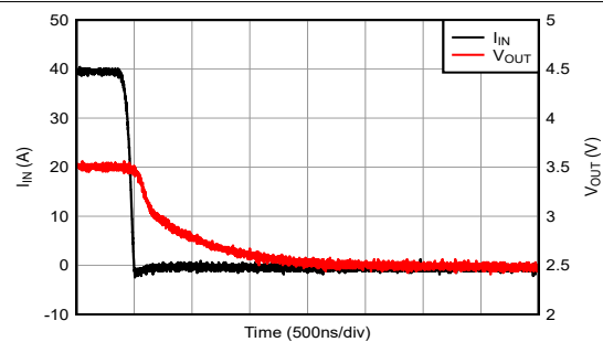
图 6-6. 电压输出阶跃响应 (下降)
