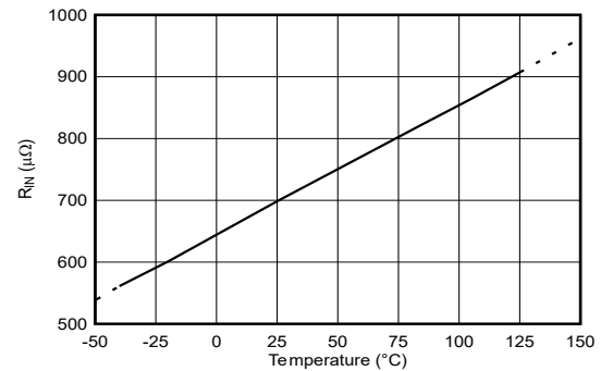
图 6-12. 输入导体电阻与温度间的关系
