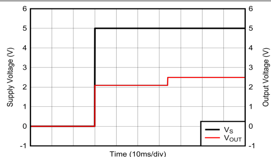
图 6-8. 启动瞬态响应
