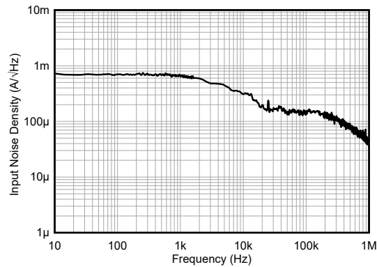
图 6-11. 输入基准电压噪声密度与频率间的关系
