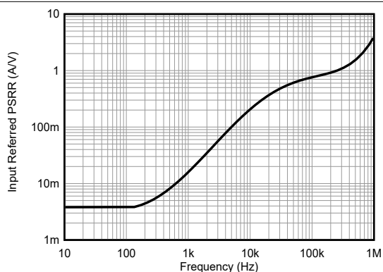
图 6-3. PSRR 与频率间的关系
