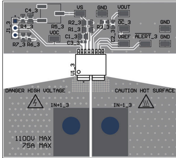
图 9-5. 建议的电路板布局布线
