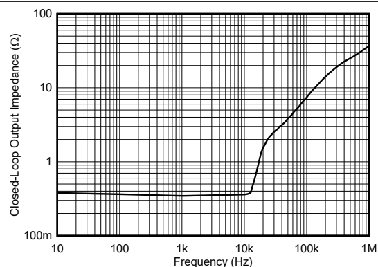
图 6-4. 输出阻抗与频率间的关系
