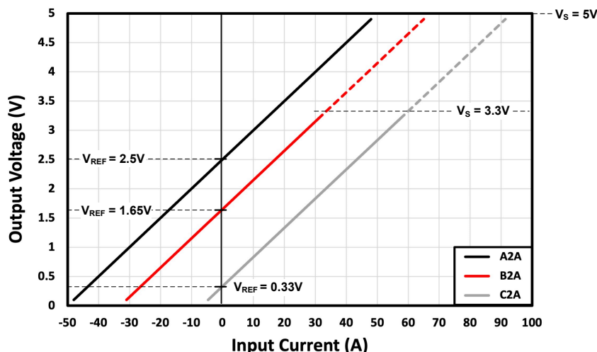
图 8-3. TMCS11xxx2A-Q1 的输出电压与输入电流之间的关系
