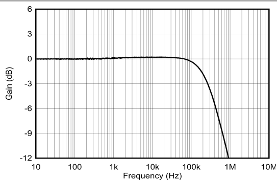
图 6-1. 灵敏度与频率间的关系 (所有增益都归一化为 1Hz)
