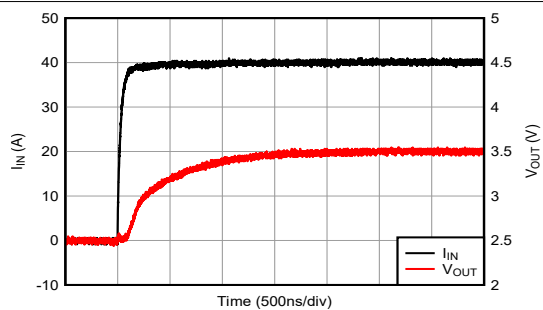
图 6-5. 电压输出阶跃响应 (上升)
