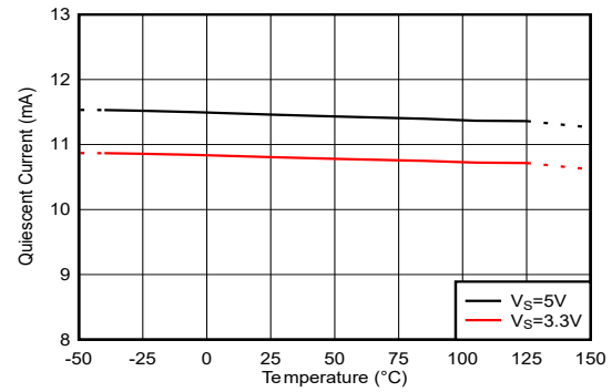
图 6-10. 静态电流与温度间的关系
