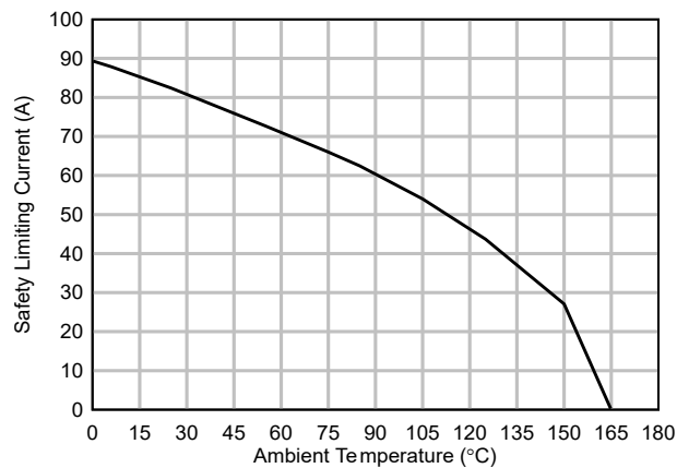
图 6-13. 安全限制电流的热降额曲线，侧 1
