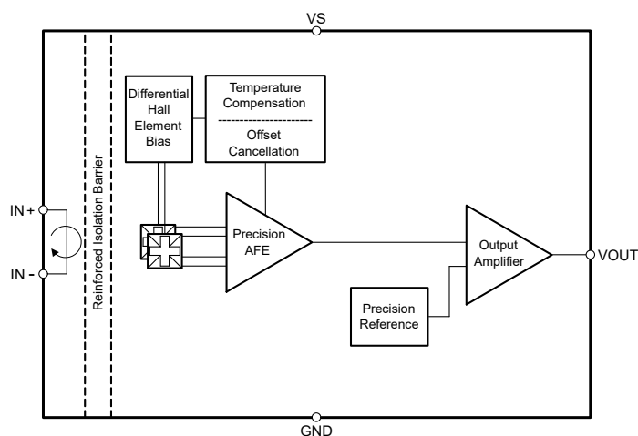
图 8-1. 功能方框图
