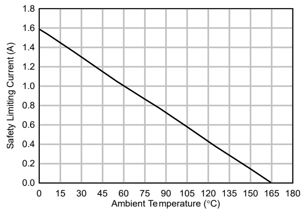
图 6-14. 安全限制电流的热降额曲线，侧 2
