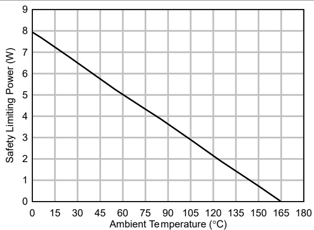
图 6-15. 安全限制功率的热降额曲线
