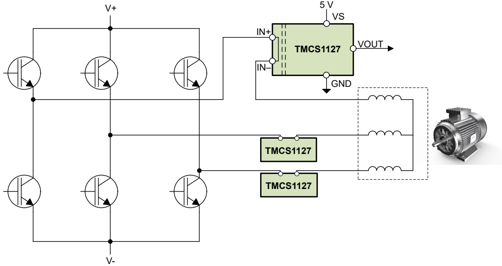
图 9-2. 内嵌式电机相电流检测
