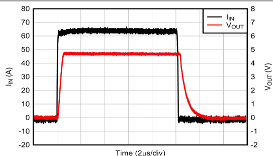
图 6-7. 电流过载响应
