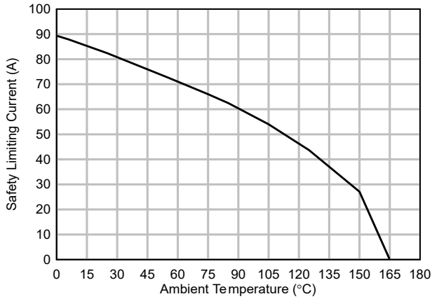
图 6-23. 安全限制电流的热降额曲线，侧 1
