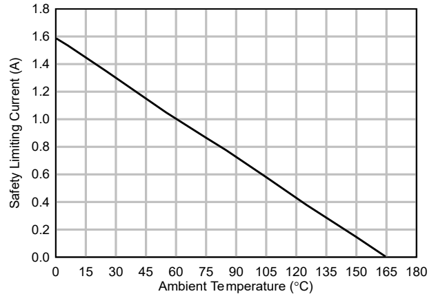
图 6-24. 安全限制电流的热降额曲线，侧 2
