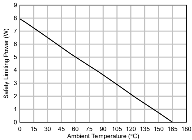
图 6-25. 安全限制功率的热降额曲线
