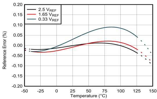
图 6-3. 基准误差与温度间的关系
