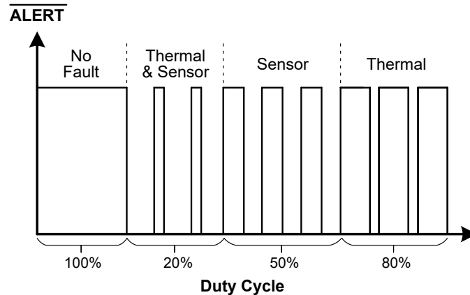
图 8-9. 传感器诊断波形
