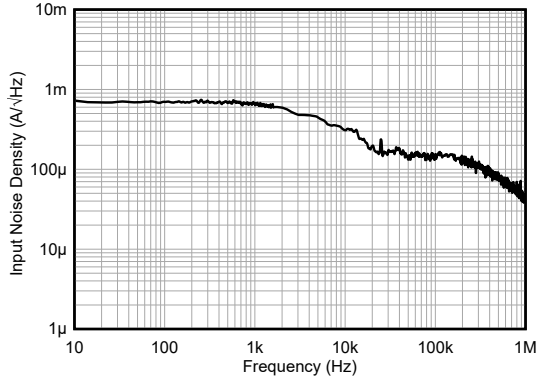
图 6-21. 输入基准电压噪声密度与频率间的关系
