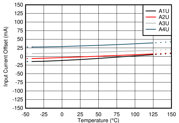
图 8-3. 整个温度范围内的失调误差漂移 (U 型号)
