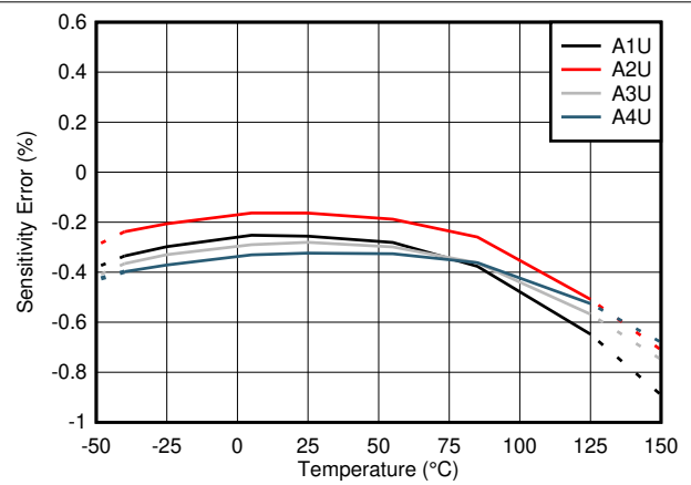
图 6-2. TMCS1101AxU 灵敏度误差与温度间的关系
