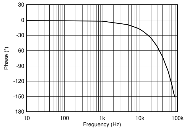
图 6-18. 相位与频率间的关系 (所有增益)
