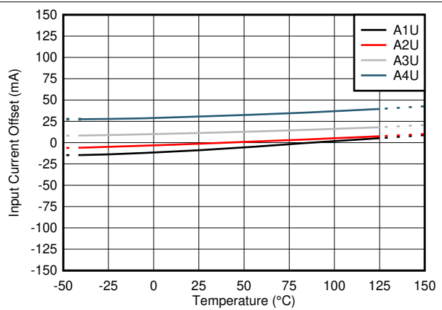
图 6-4. TMCS1101AxU 输入失调电流与温度间的关系
