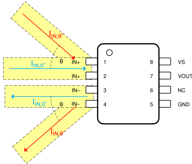
图 9-3. 输入电流引线产生的磁场
