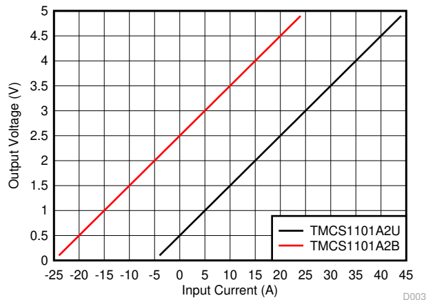
图 8-14. TMCS1101A2B 和 TMCS1101A2U 输出电压与输入电流的关系
