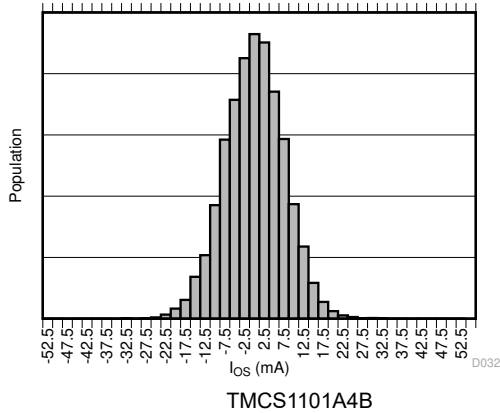
图 6-15. 输入偏移电流产生分布图
