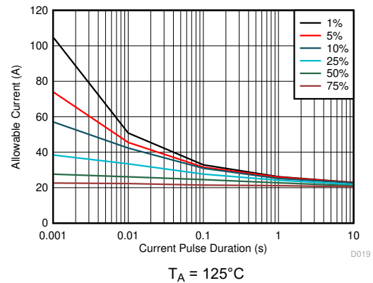
图 7-9. 最大重复脉冲电流与脉冲持续时间间的关系
