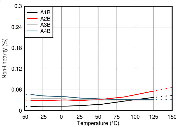
图 6-5. 非线性与温度间的关系
