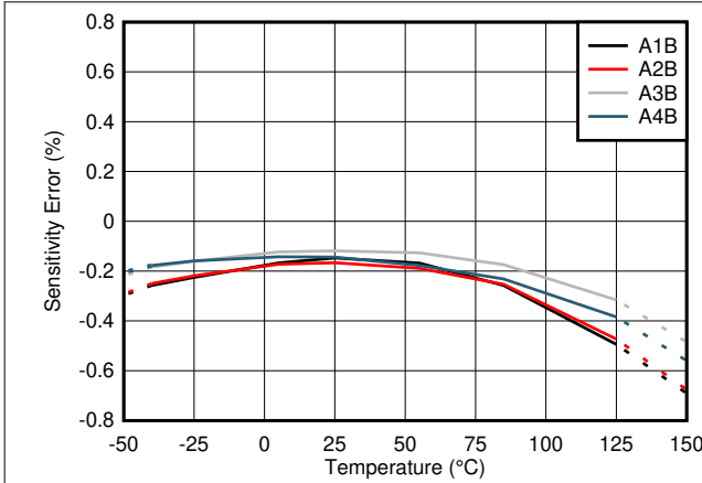
图 6-1. TMCS1101AxB 灵敏度误差与温度间的关系
