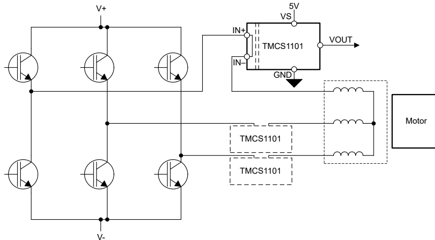
图 9-2. 内嵌式电机相电流检测
