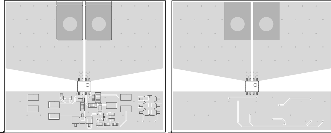
图 9-5. 建议的板顶部 ( 左侧 ) 和底部 ( 右侧 ) 平面布局
