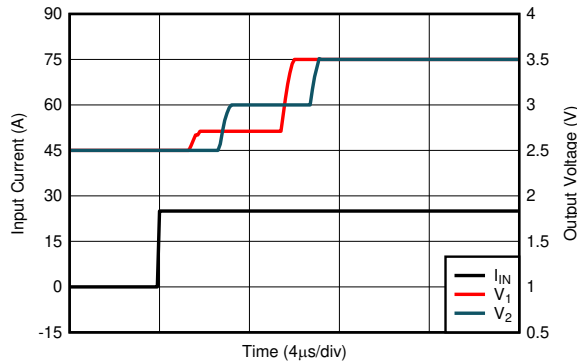
图 6-23. 电压输出阶跃 (上升)
