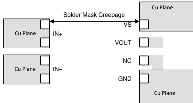
图 9-4. 满足系统爬电要求的布局
