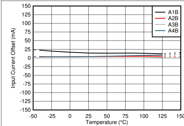
图 6-3. TMCS1101AxB 输入失调电流与温度间的关系
