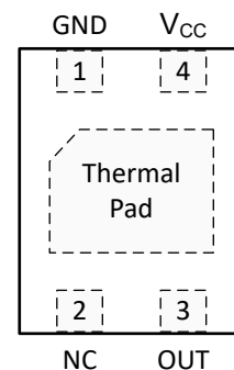
图 6-2. DMR 封装 4 引脚 X2SON 顶视图
