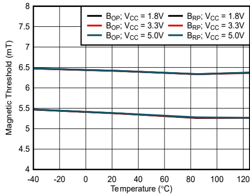
图 6-3. 6.3mT B OP : 阈值与温度间的关系
