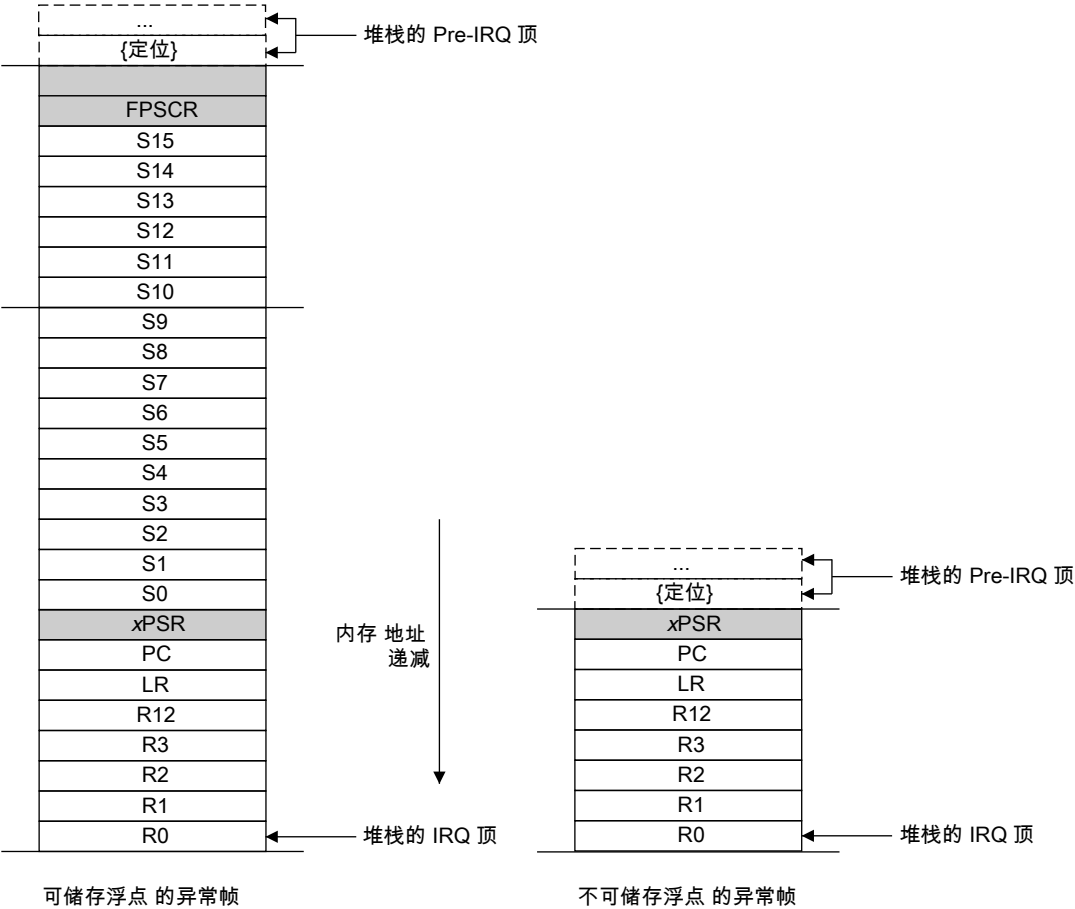
图 2-7. 异常堆栈框
