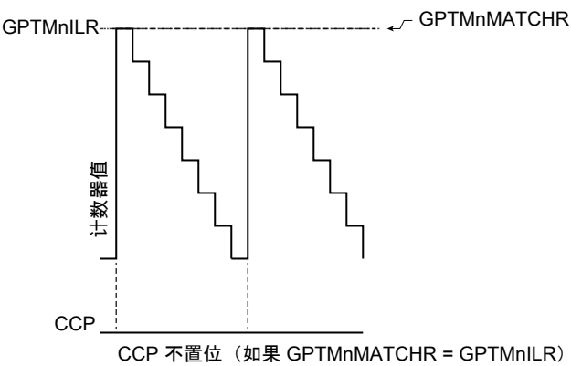
图 10-7. CCP 输出，GPTMTnMATCHR = GPTMTnILR
