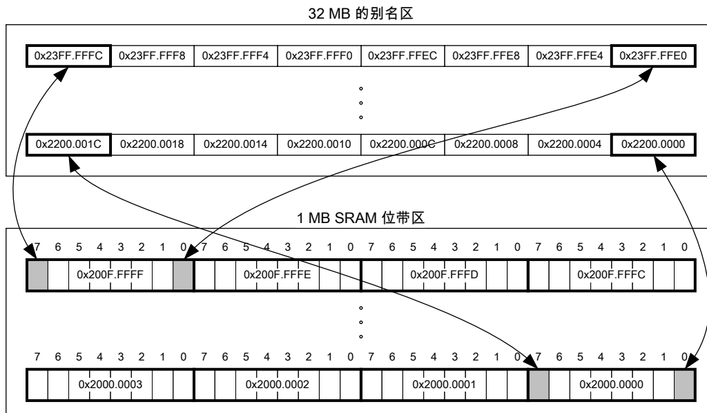
图 2-4. 位带映射
