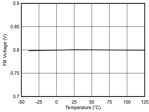
图 5-1. 反馈电压
