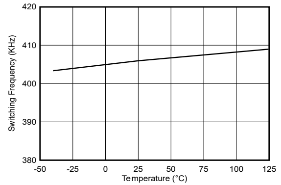
图 5-6. f_{sw} 400kHz
