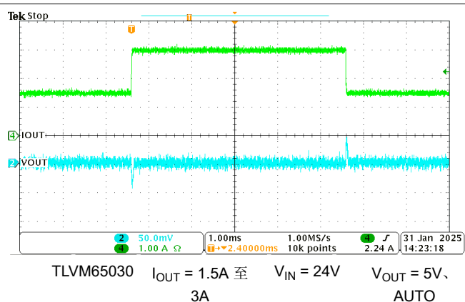
图 7-6. 负载瞬态 (50% 至 100%)
