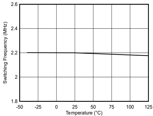
图 5-5. f_{sw} 2.2MHz
