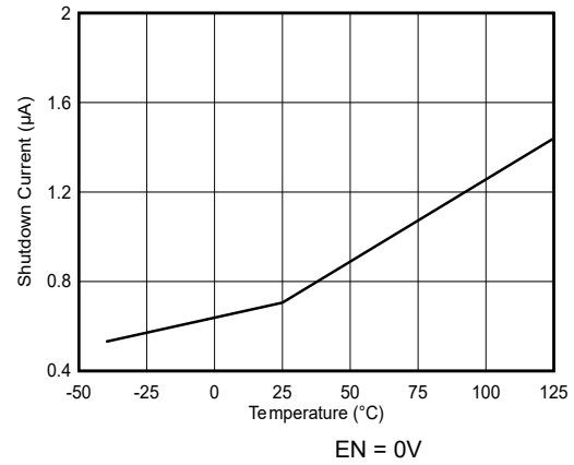
图 5-2. 关断输入电流
