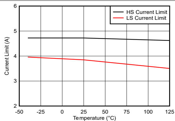
图 5-8. 电流限值
