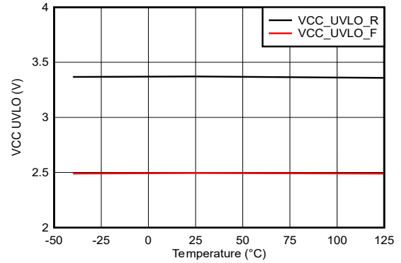
图 5-4. V_{CC} UVLO
