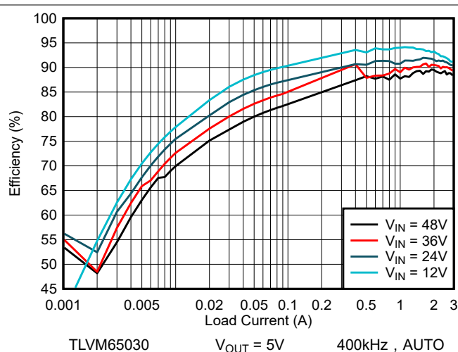
图 7-4. 效率
