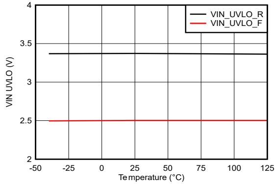
图 5-3. 启用 UVLO
