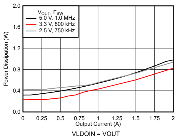
图 7-12. 功率耗散
