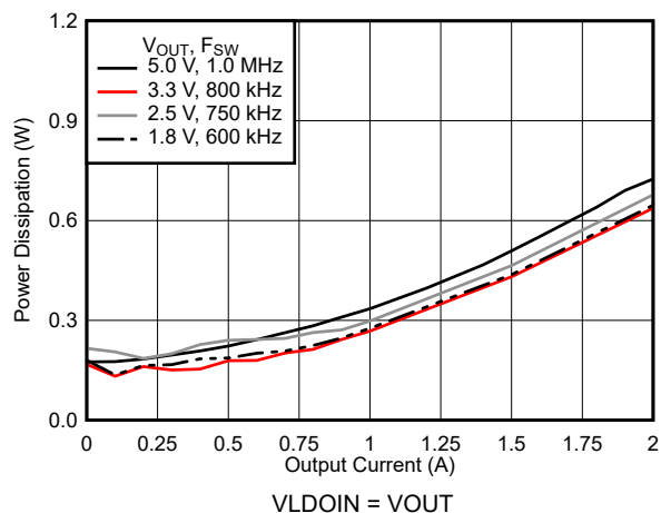
图 7-8. 功率耗散
