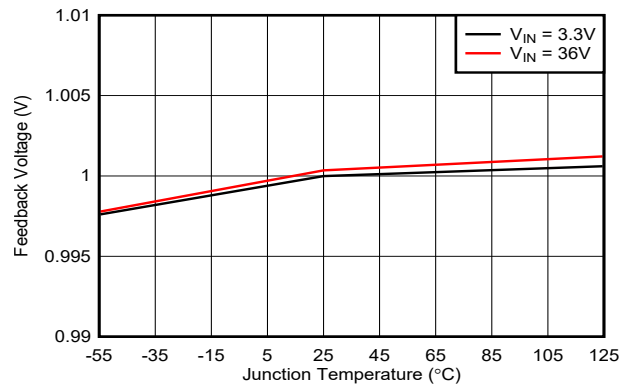
图 7-2. 反馈电压
