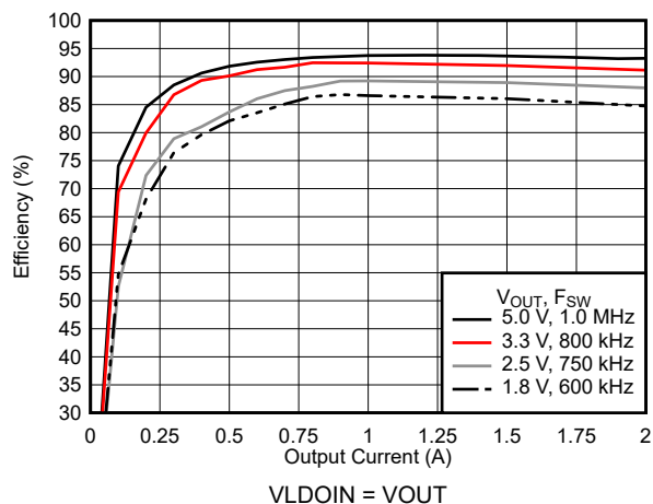
图 7-7. 效率
