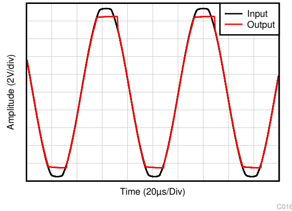
图 7-4. 无相位反转
