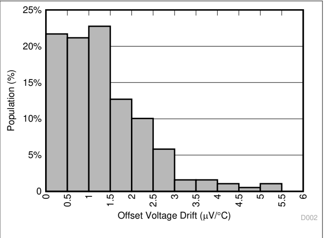
图 6-2. 失调电压漂移分布
