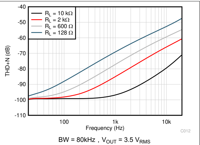
图 6-20. THD+N 比与频率间的关系
