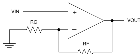
图 10-1. 原理图表示
