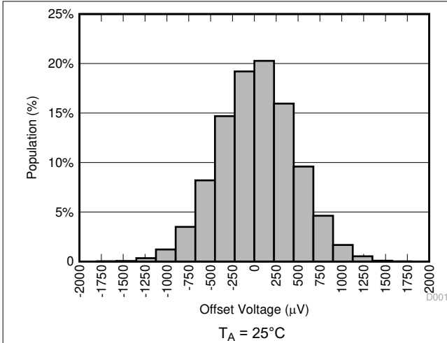
图 6-1. 失调电压生产分配
