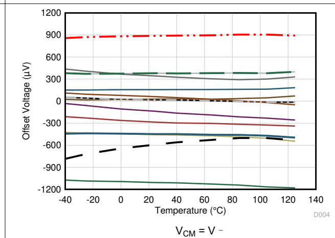
图 6-4. 失调电压与温度间的关系
