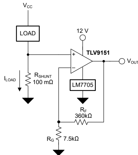
图 7-1. 低侧电流检测应用中的 TLV9151-Q1
