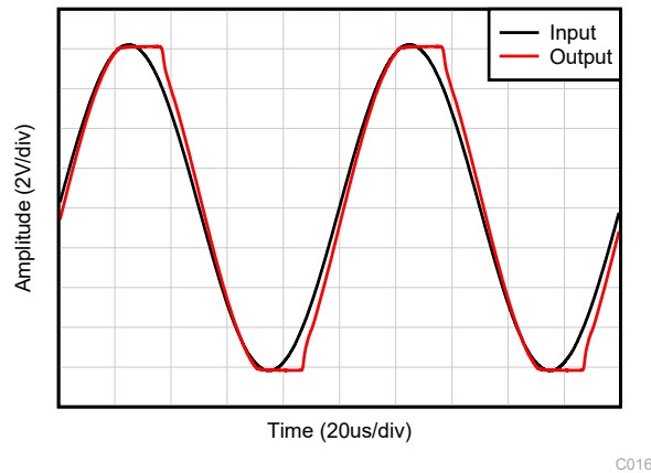
图 6-7. 无相位反转
