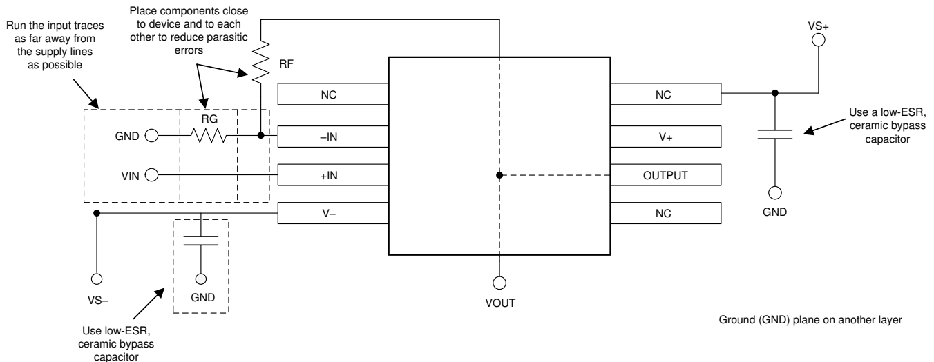
图 7-4. 同相配置的运算放大器电路板布局
