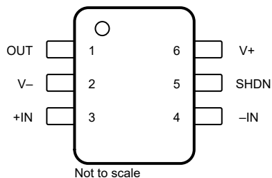
图 4-3. TLV9151S-Q1 DBV 封装， 6 引脚 SOT-23 (顶视图)
