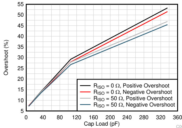
图 6-3. 小信号过冲与容性负载间的关系 ( 10mV 输出阶跃, G = 1 )
