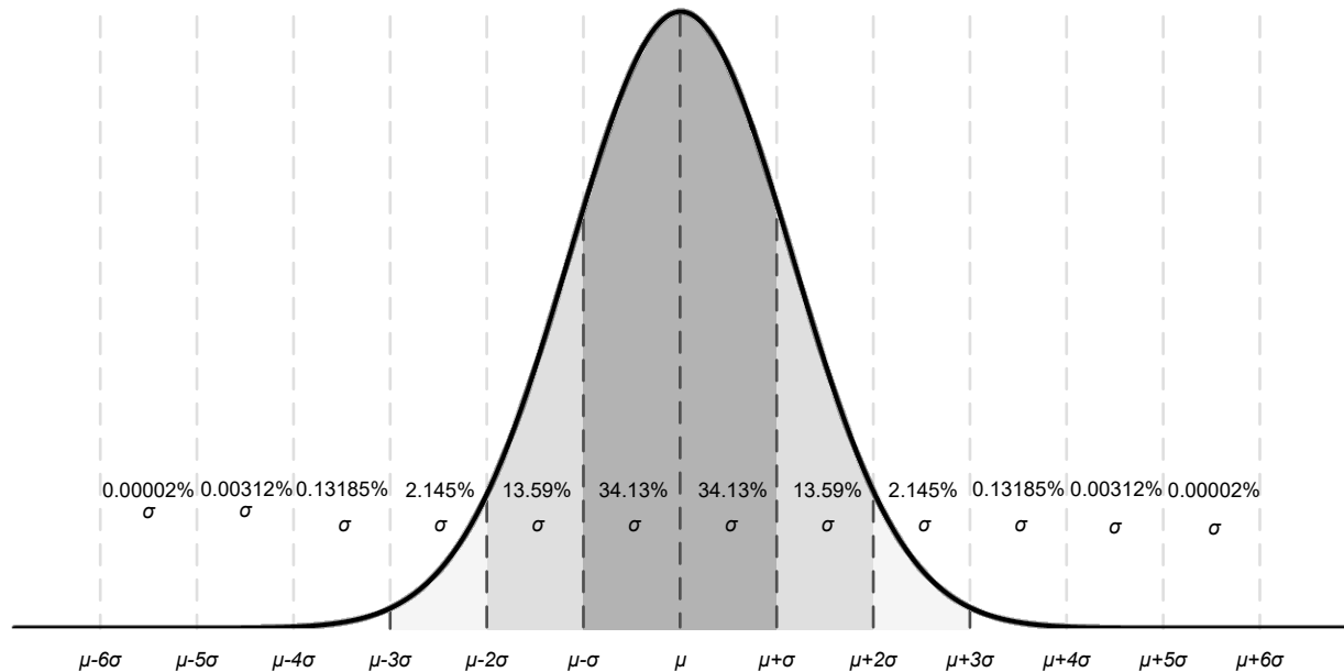
图 6-9. 理想的高斯分布
