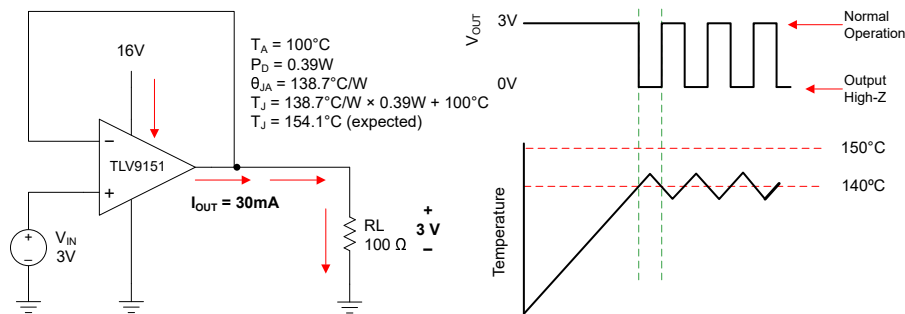
图 6-2. 过热保护
