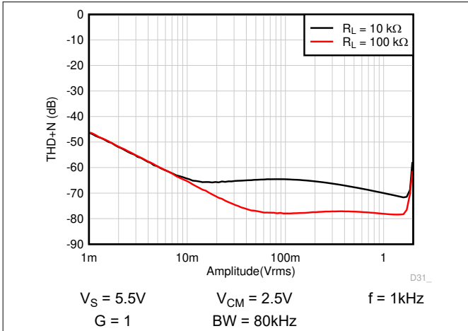
图 6-25. THD + N 与幅度间的关系
