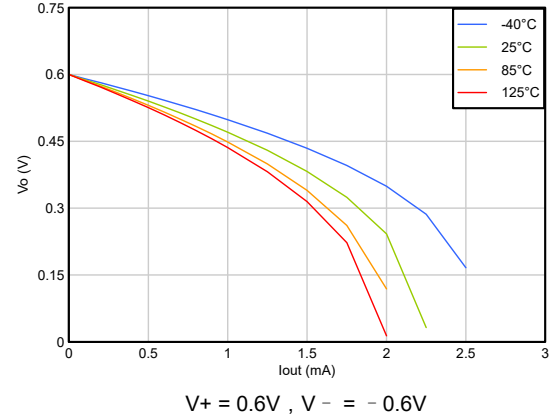
图 5-14. 输出电压与输出电流间的关系 (爪形)
