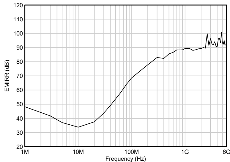
图 6-5. EMIRR 测试
