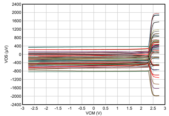
图 5-4. 失调电压与共模间的关系
