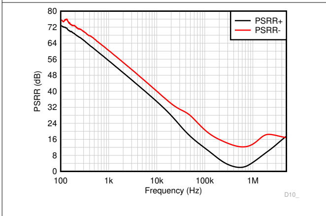
图 6-17. PSRR 与频率间的关系
