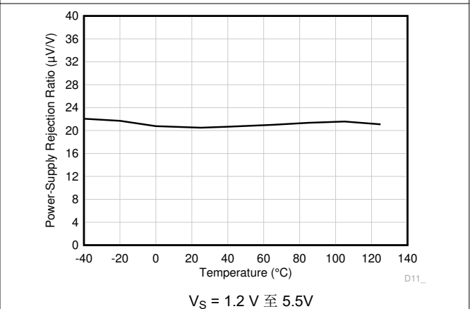
图 6-18. 直流 PSRR 与温度间的关系
