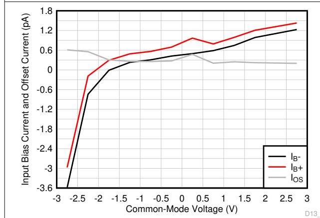
图 6-9. I_B 和 I_{OS} 与共模电压间的关系
