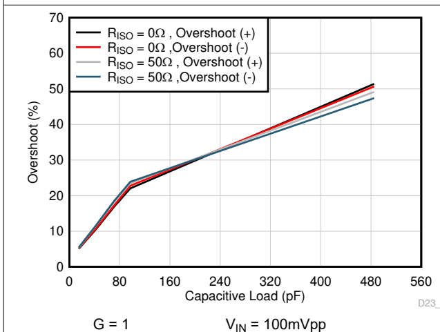
图 6-29. 小信号过冲与容性负载间的关系
