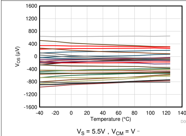
图 6-3. 输入失调电压与温度间的关系
