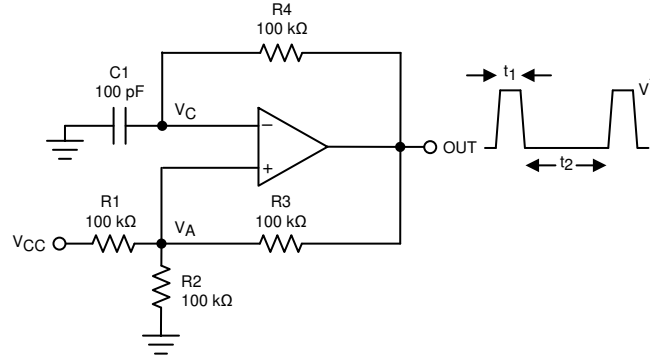
图 7-9. 方波振荡器
