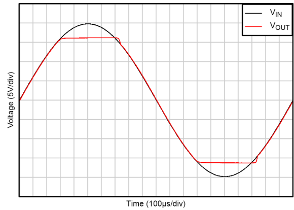
图 5-30. 无相位反转
