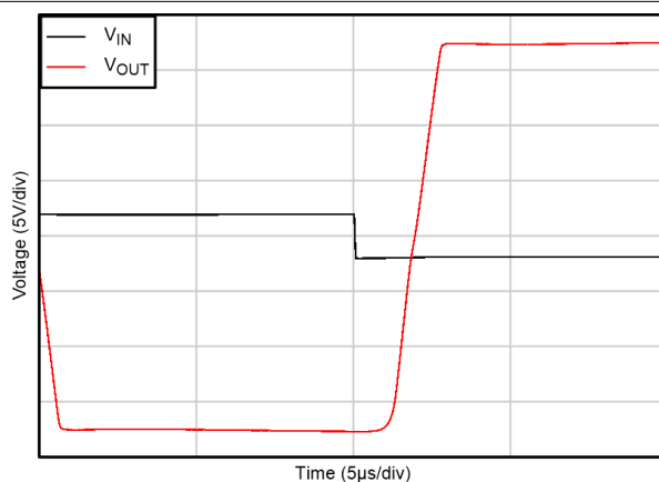
图 5-32. 负过载恢复
