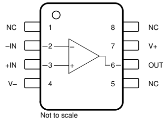
图 4-1. TLV886 : D 封装, 8 引脚 SOIC (顶视图)
