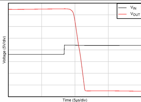
图 5-31. 正过载恢复
