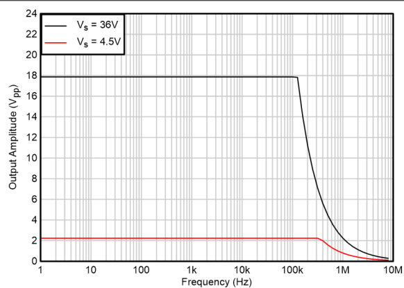
图 5-40. 最大输出电压与频率间的关系
