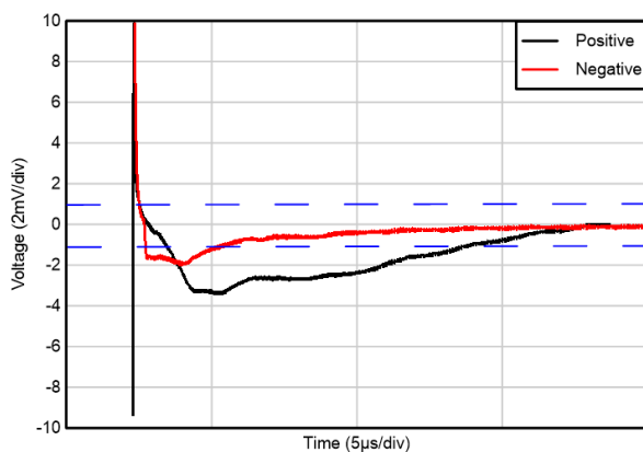
图 5-38. 趋稳时间
