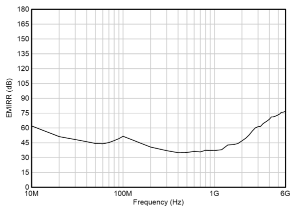
图 5-41. EMIRR 与频率间的关系
