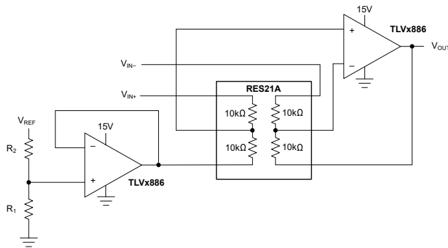
图 7-6. 差分放大器
