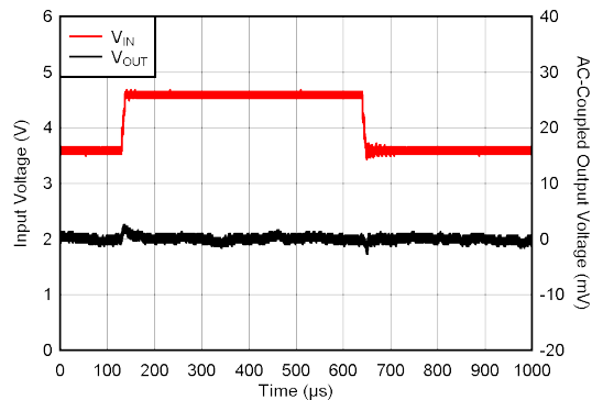
图 5-13. 线路瞬态
