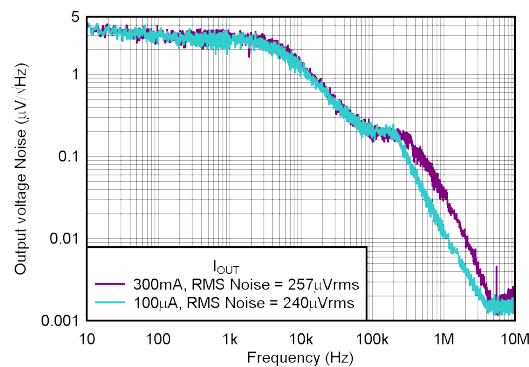
图 5-17. 噪声
