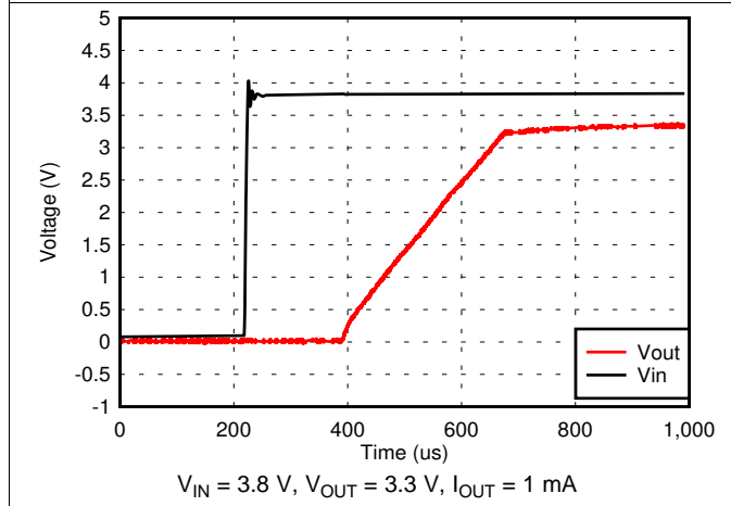
图 23. V_{IN} Power-Up
