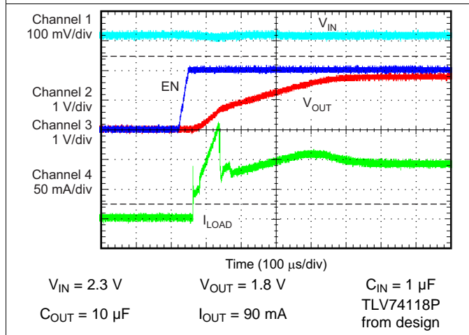
图 21. Start-Up With EN
