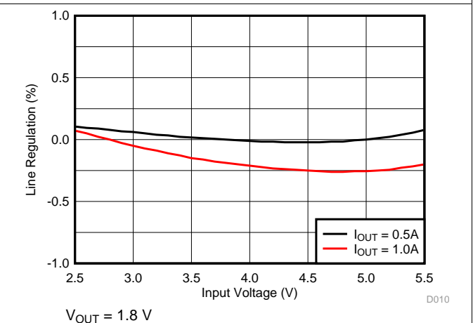
图 11. Line Regulation
