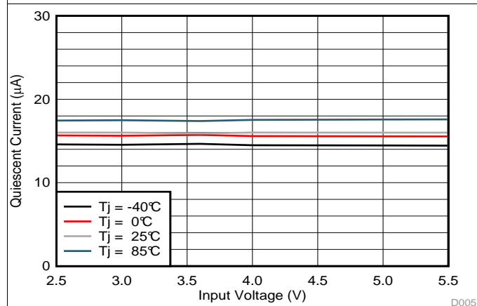
图 3. Quiescent Current
