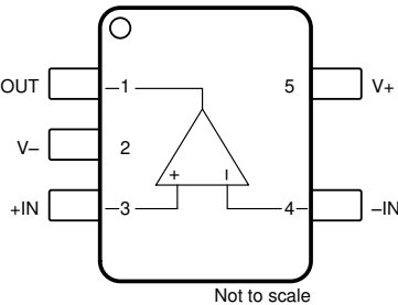
图 4-2. TLV888：DBV 封装，5 引脚 SOT-23（顶视图）
