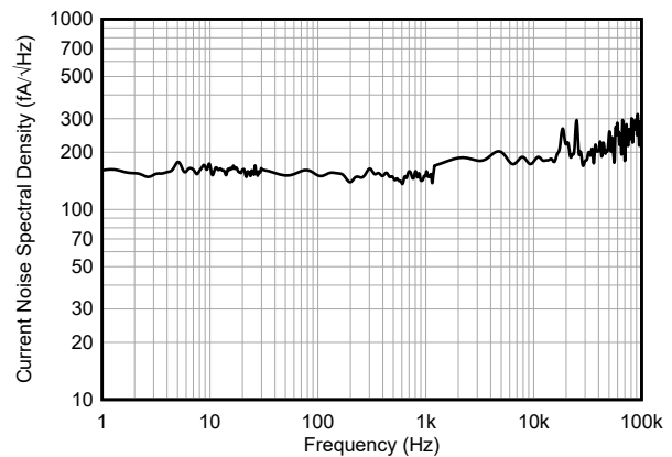
图 5-22. 输入电流噪声频谱密度与频率间的关系
