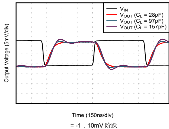
图 5-34. 小信号阶跃响应
