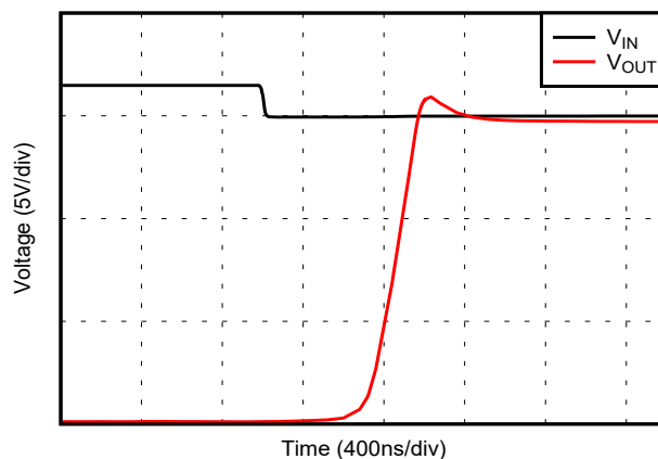
图 5-32. 负过载恢复
