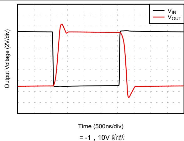
图 5-36. 大信号阶跃响应
