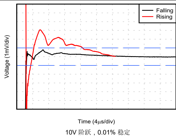
图 5-38. 稳定时间
