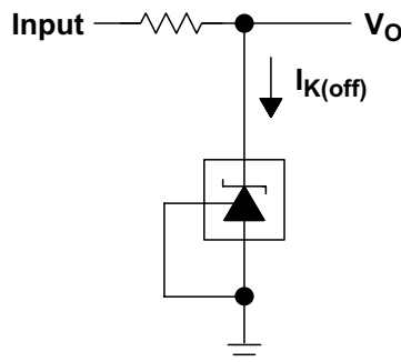
图 6-3. 针对 I_{K(off)} 的测试电路
