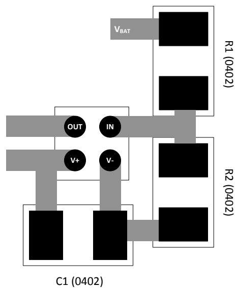
图 11-1. Layout Example
