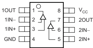
图 5-3. TLV3702 D、DGK 或 P 封装 8 引脚 SOIC、VSSOP 或 PDIP 顶视图
