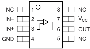
图 5-2. TLV3701 D 或 P 封装 8 引脚 SOIC 或 PDIP 顶视图
