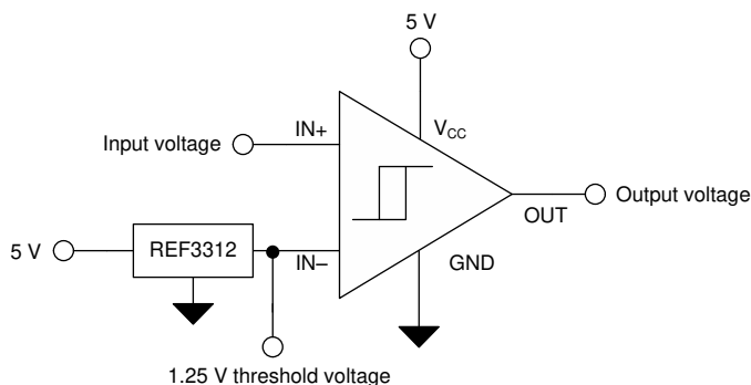
图 8-1. 1.25V 阈值检测器
